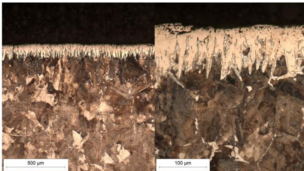
Slika 28. Mikrostruktura boriranih uzoraka pod povećanjem 50x (lijevo) i 200x (desno)
