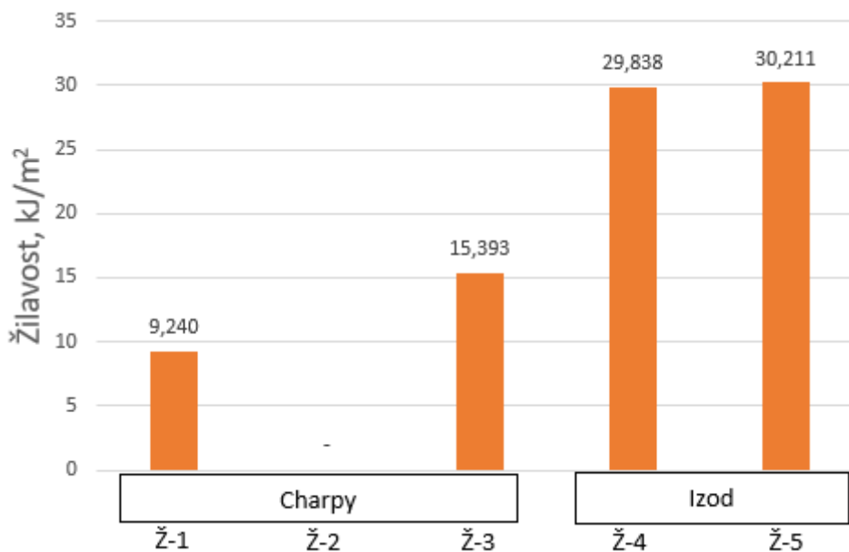
Slika 5.17. Srednje vrijednosti žilavosti po Charpyu i Izodu
