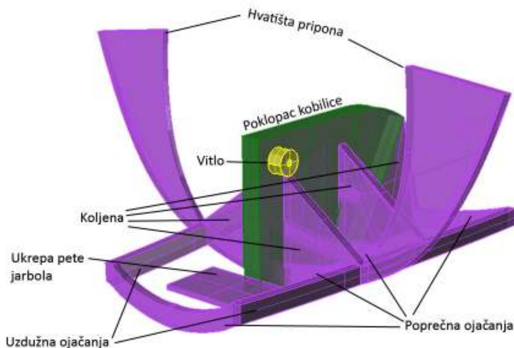
Slika 6.1. Roštilj kobilice
