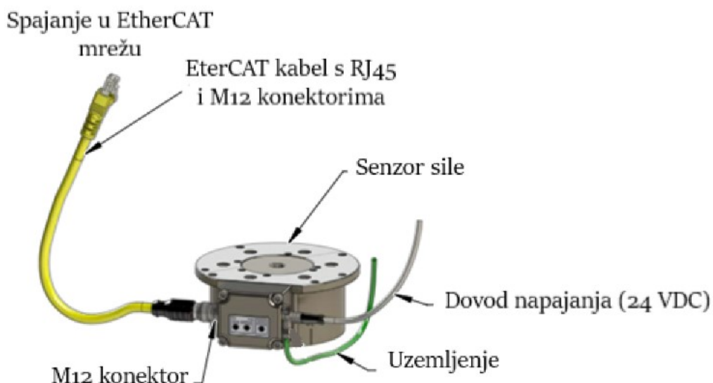
Slika 5-9. Način spajanja mjerne ćelije, prilagođeno iz [24]
