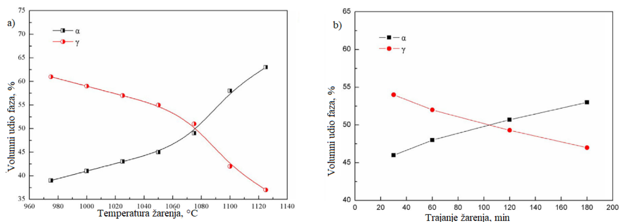
Slika 22. Dijagram promjene udjela faza s porastom temperature žarenja[29]
