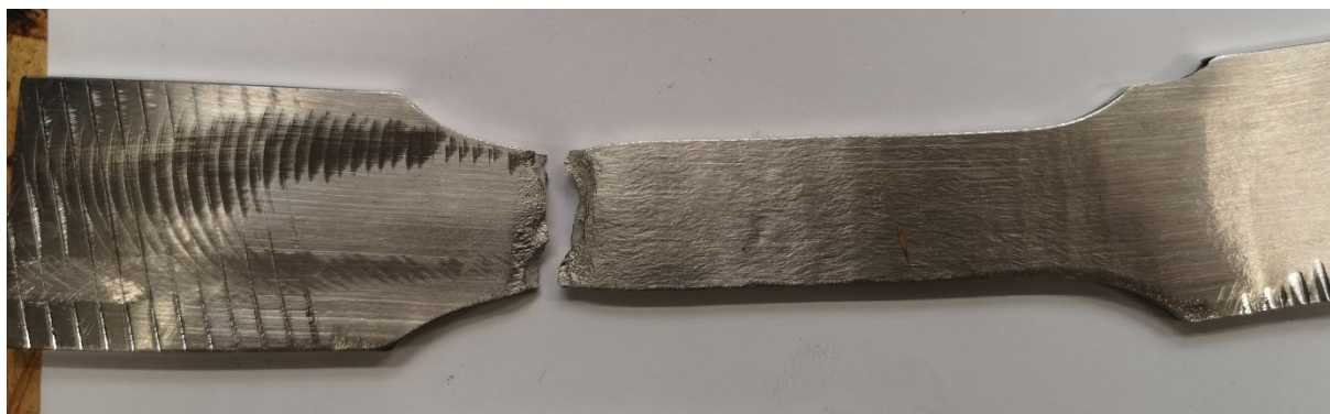
Slika 52. Puknuće epruvete 2V na mjestu zavora
