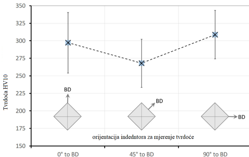
Slika 13. Anizotropnost tvrdoće (BD-smjer nanošenja slojeva)[24]
