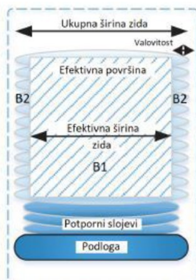
Slika 5. Efektivna širina zida izrađenog WAAM postupkom [12]
