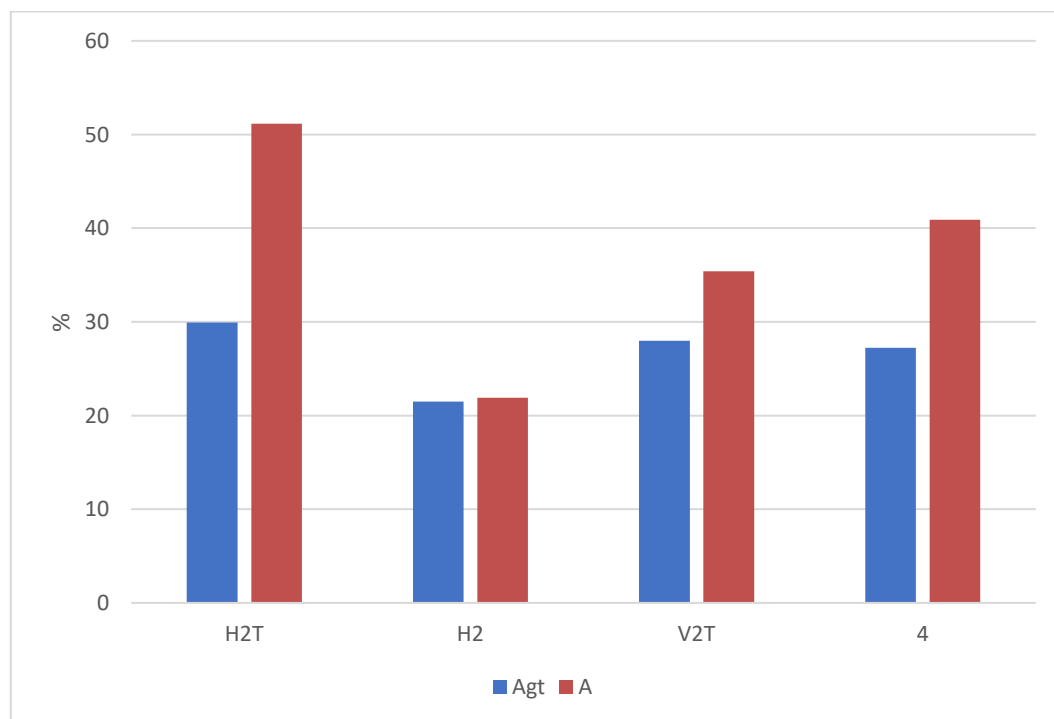
Slika 89. Usporedba istezljivosti pri vlačnoj čvrstoći
