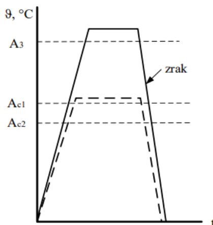
Slika 20. Dijagram kontinuiranog hlađenja kod normalizacije čelika [3]
