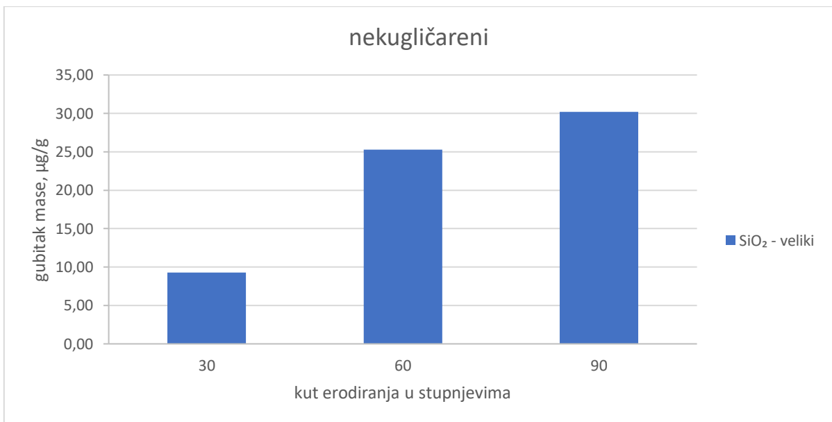
Slika 182: Gubitak mase po kutu erodiranja, nekugličarenog, neobrađenog ADI 240, uslijed erodiranja erozivom oznake SiO 2 - veliki
