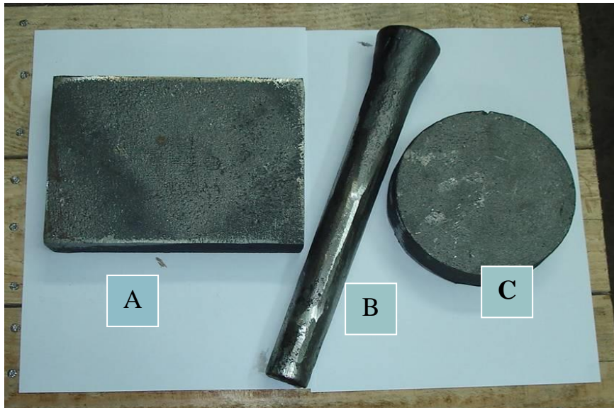
Slika 55: Odljevci EN-GJS-600-3 [45]
