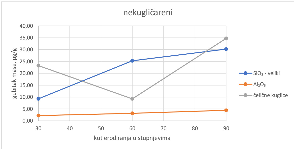
Slika 181: Gubitak mase nekugličarenog, neobrađenog ADI 240 po kutu erodiranja različitim erozivima
