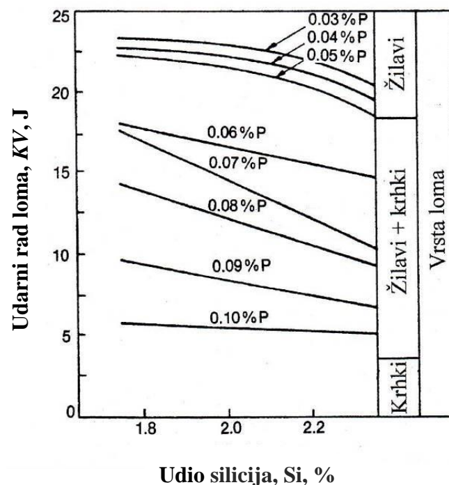
Slika 12: Utjecaj fosfora i silicija na udarni rad loma [10]
