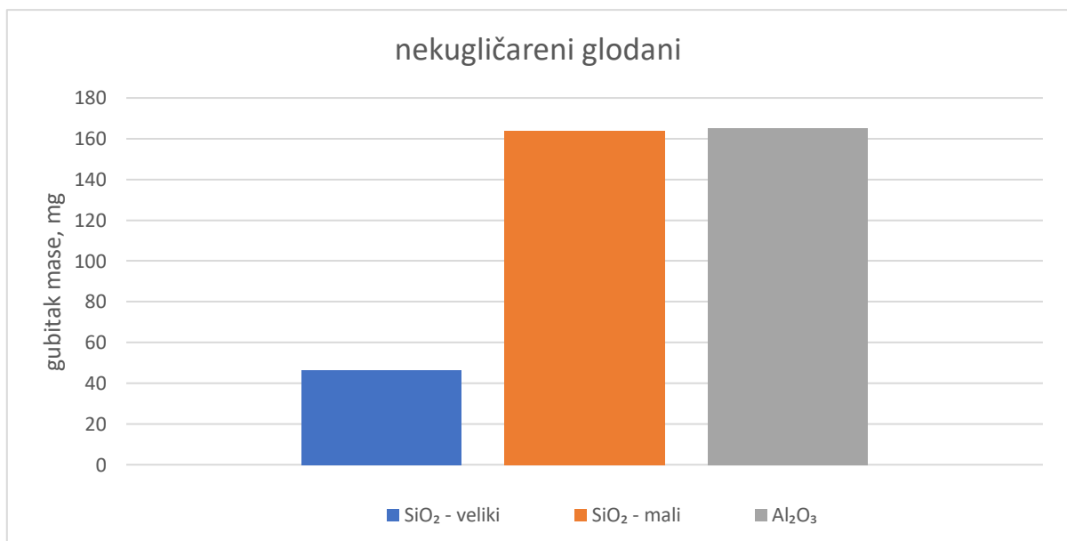
Slika 156: Prosječan gubitak mase ADI 240, za tri ciklusa abrazije različitim abrazivima
