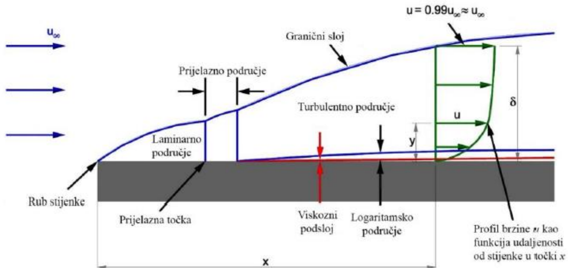
Slika 5. Granični sloj kod strujanja viskoznog fluida uz čvrstu stijenu [20]
