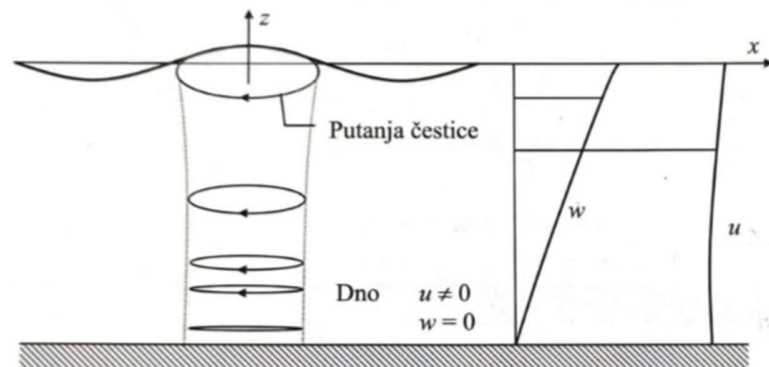
Slika 3 Trajektorije čestica vala u fluidu ograničene dubine [1]
