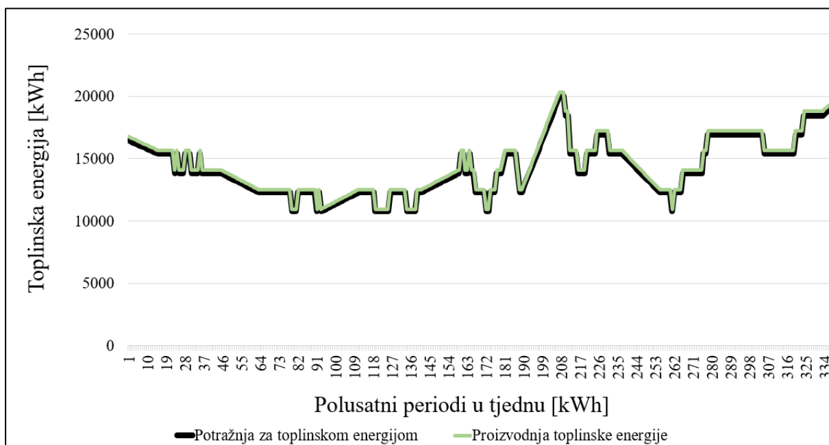
Slika 30. Potražnja i proizvodnja toplinske energije tijekom karakterističnog zimskog tjedna - Calliope
