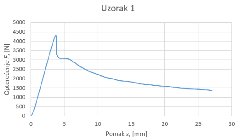
Slika 53. Dijagram sila-pomak 1. uzorka
