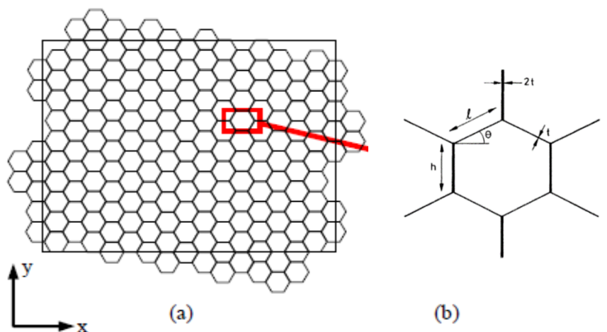
Slika 13. Ćelija saća
