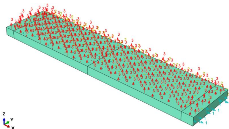
Slika 27. Definiranje orijentacije materijala
