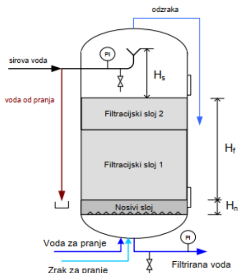
Slika 6 Tlačni filter [3]
