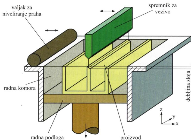
Slika 10. - Načelo 3DP postupka [1]
