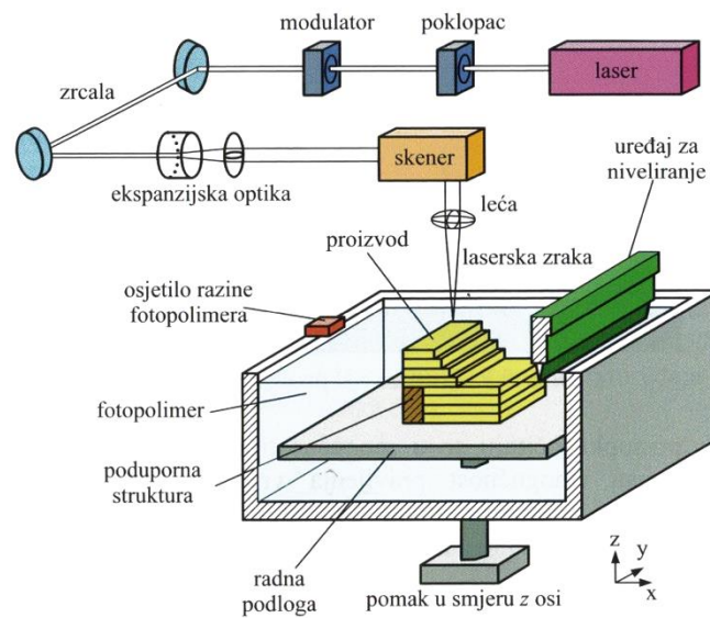
Slika 6. - Načelo SL postupka [1]
