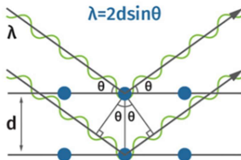
Slika 26. Bragg-ov zakon [19]
