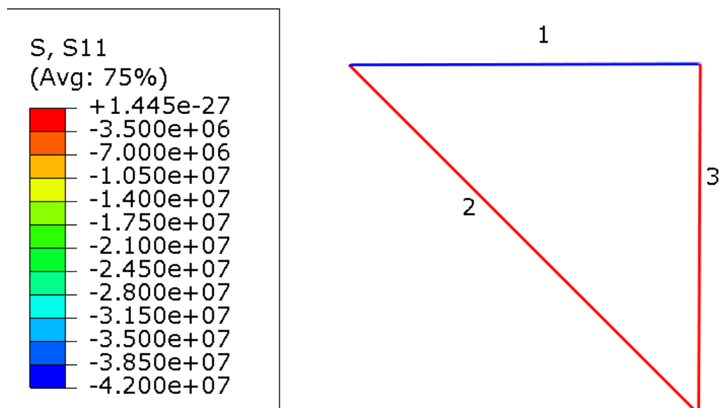
Slika 25. Raspodjela napreznja po štapnoj konstrukciji
