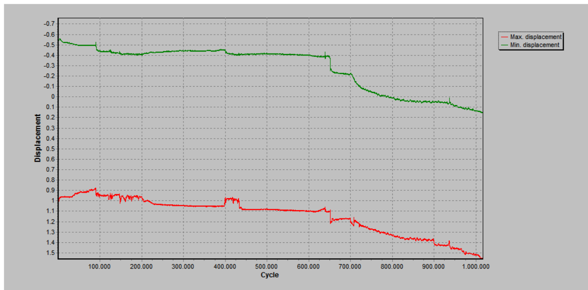
Slika 5.2 Dijagram pomak-ciklus
