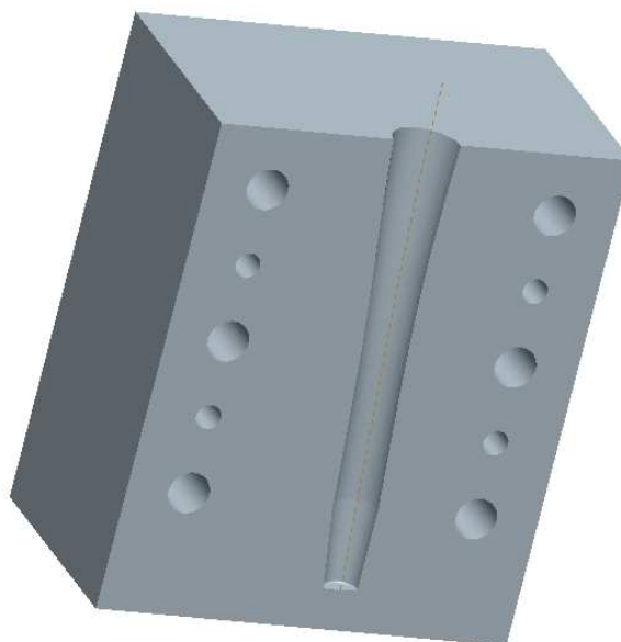
Slika 4.3 CAD model pomičnog dijela prihвата
