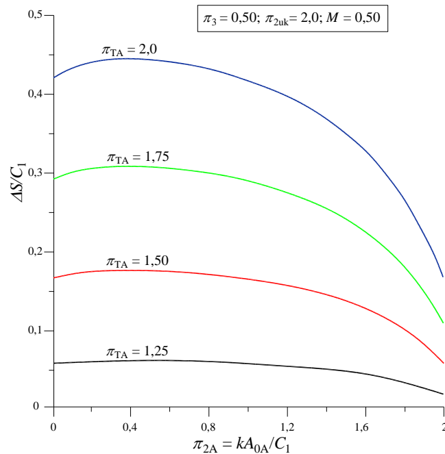
Slika 67. Zavisnost bezdimenzijske generirane entropije umreženog rekuperatora
