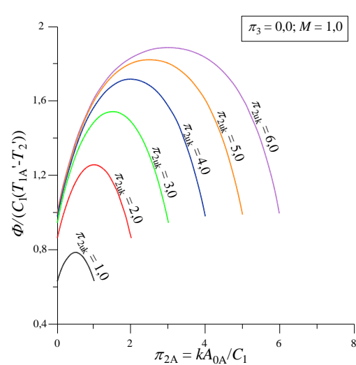
Slika 17. Zavisnost bezdimenzijskog toplinskog toka umreženog rekuperatora o \pi_{2A} i \pi_{2uk} uz \pi_3 = 0,0 ; M = 1,0
