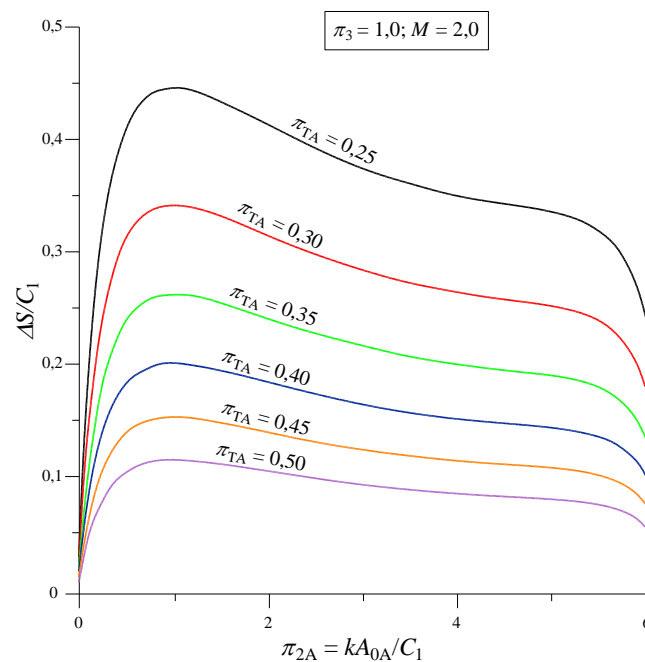
Slika 79. Zavisnost bezdimenzijske generirane entropije umreženog rekuperatora o \pi_{2A} i \pi_{TA} = 0,25; 0,3; 0,35; 0,40; 0,45 i 0,50 uz \pi_3 = 1,0; \pi_{2uk} = 6,0 i M = 2,0
