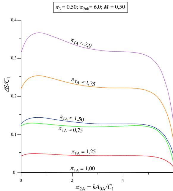
Slika 61. Zavisnost bezdimenzijske generirane entropije umreženog rekuperatora
