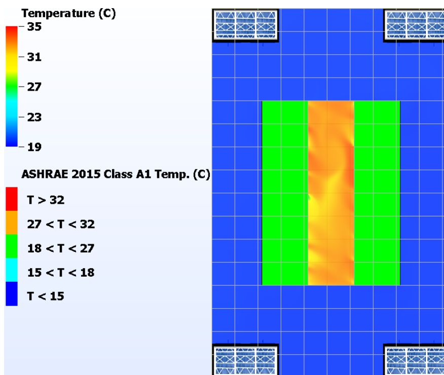
Slika 52. IT ormari grupirani prema najvišoj temperaturi na ulazu u servere u tloctu zakrenutom za 90°
