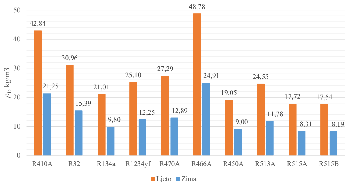
Slika 46 – Gustoća radne tvari na usisu u kompresor pri projektним uvjetima
