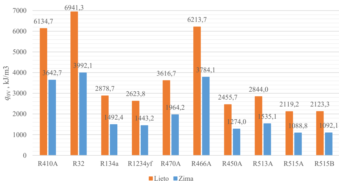
Slika 47 – Volumetrički rashladni učin pri projektним uvjetima
