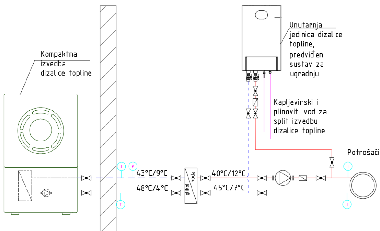
Slika 28. Shema spajanja dizalica topline sa sustavom grijanja i hlađenja
