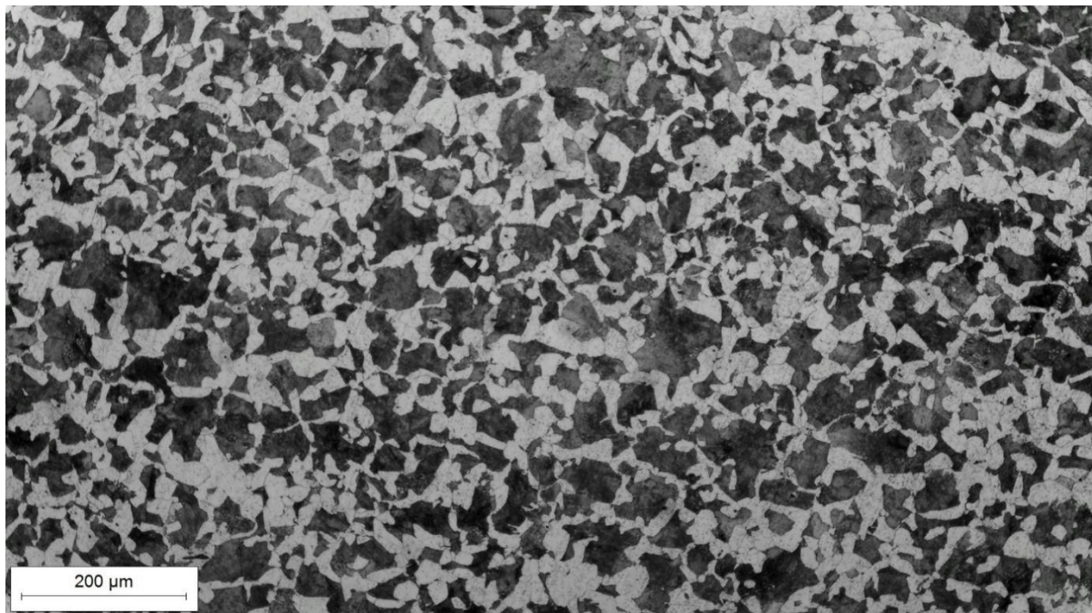
Slika 37. Mikrostruktura zuba analiziranog zupčanika snimljena pri povećanju 100×.
