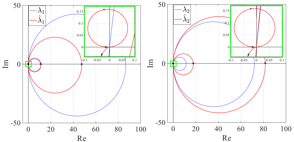
Slika 4.5 Nyquistove konture vlastitih vrijednosti matrice prijenosnih funkcija između mjernih i pogonskih članova: model s uključenom dinamikom mjernih i pogonskih članova – crveno, model bez dinamike mjernih i pogonskih članova – plavo (crni kružići prikazuju vlastite frekvencije sustava, crni dijaman prikazuje graničnu frekvenciju kruga elektrodinamičkih pogonskih članova, crni kvadratić frekvenciju prelaska konture preko negativne realne osi, a crni "×" vlastitu frekvenciju mjernih članova)
