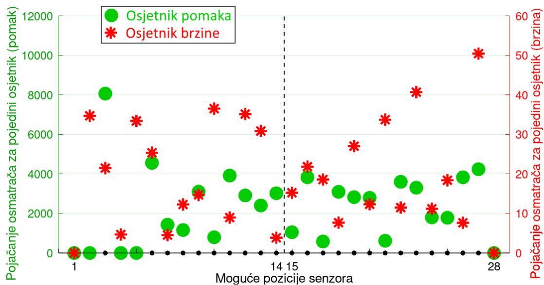
Slika 11. Pojaćanje osmatrača osjetnika za \alpha_2 = 0.00007, T_3
