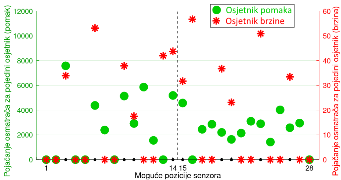
Slika 12. Pojaćanje osmatrača osjetnika za \alpha_2 = 0.00028, T_4
