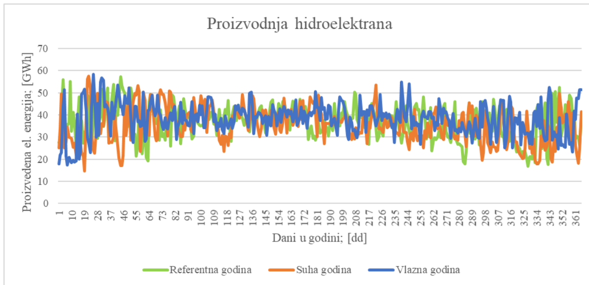
Slika 34 Proizvodnja hidroelektrana s obzirom na hidrološke uvjete – Dispa – SET MTHC model – 2050 – S1
