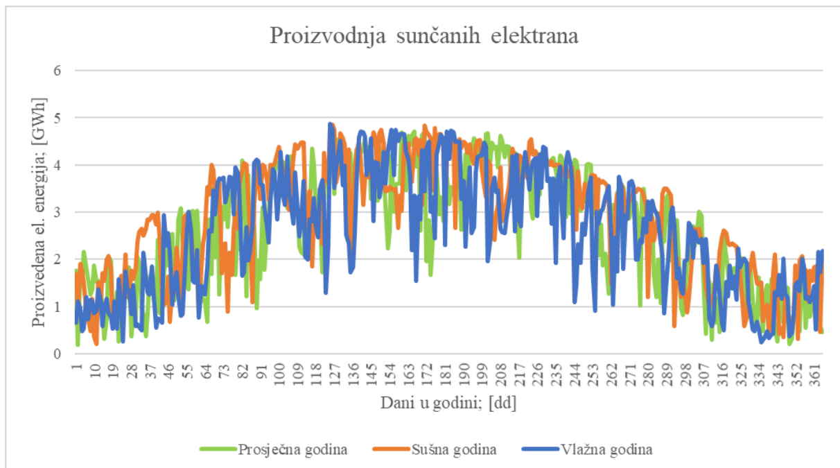
Slika 40 Proizvodnja sunčanih elektrana – Dispa – SET MTHC model – 2030 – S2
