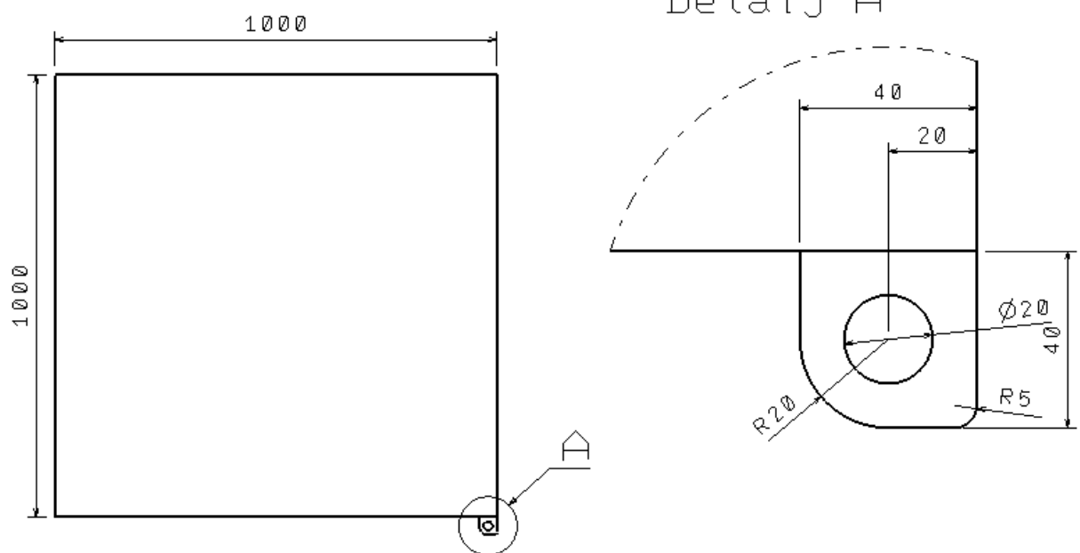
Detalj A
