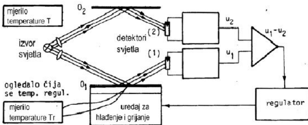
Slika 2. Mjerenje relativne vlažnosti pomoću rosišta
