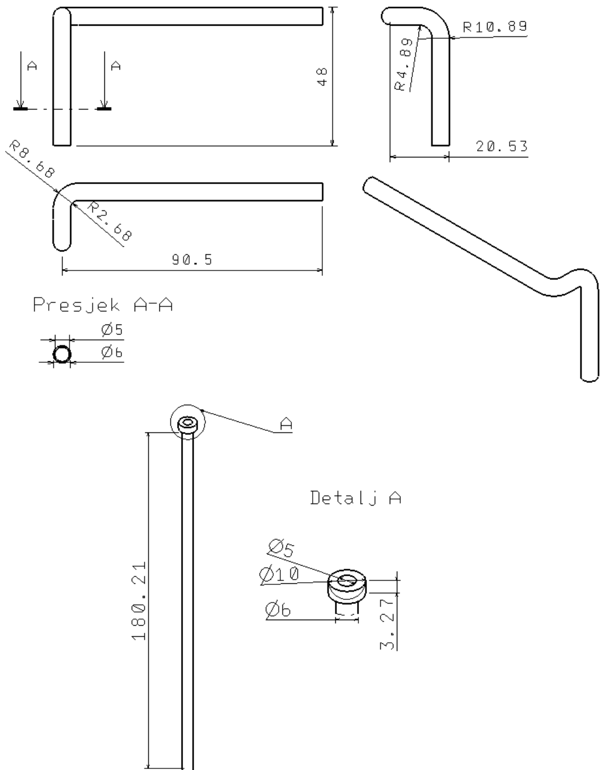
Slika 40. Cijev ispusta saturatora
