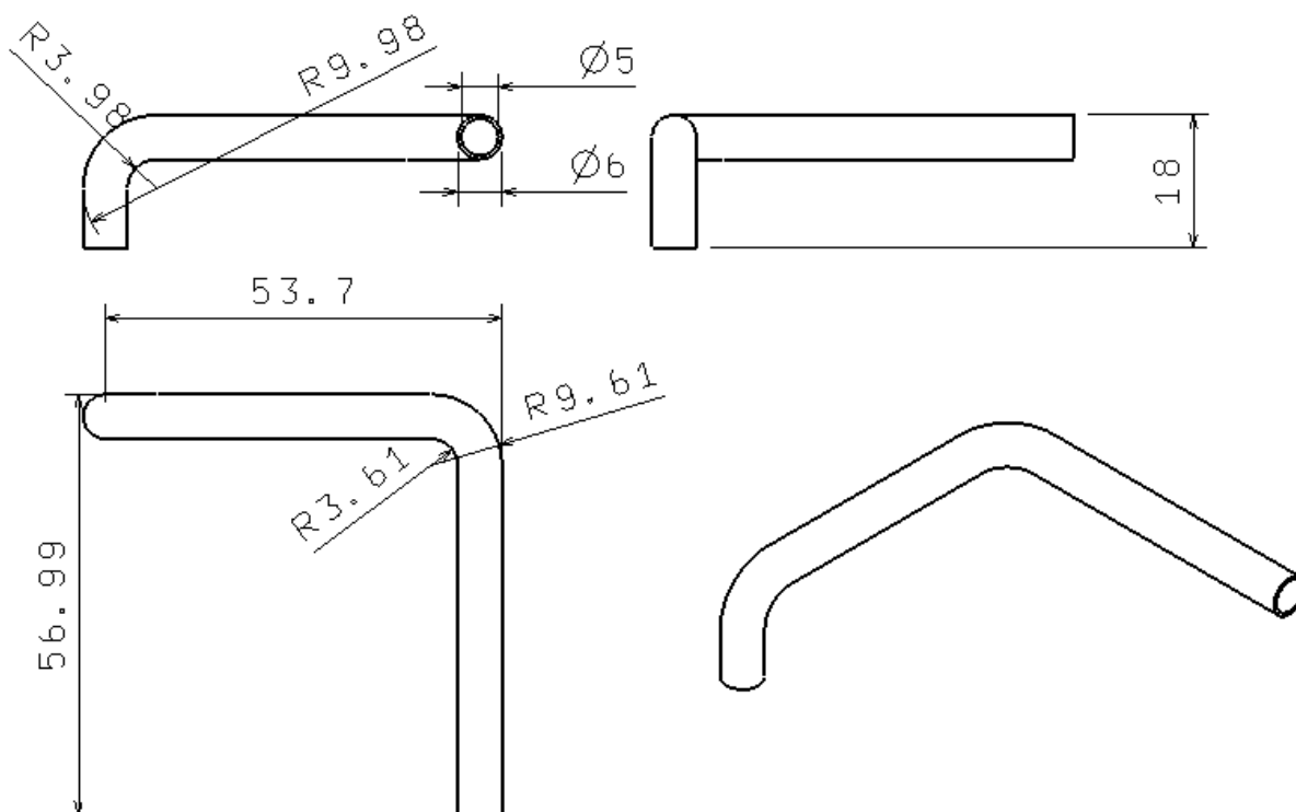
Slika 39. Cijev ispusta predsaturatora
