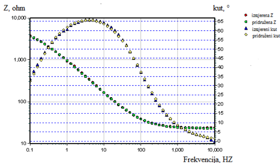
Slika 34 Bodeov dijagram s pridruženim vrijednostima
