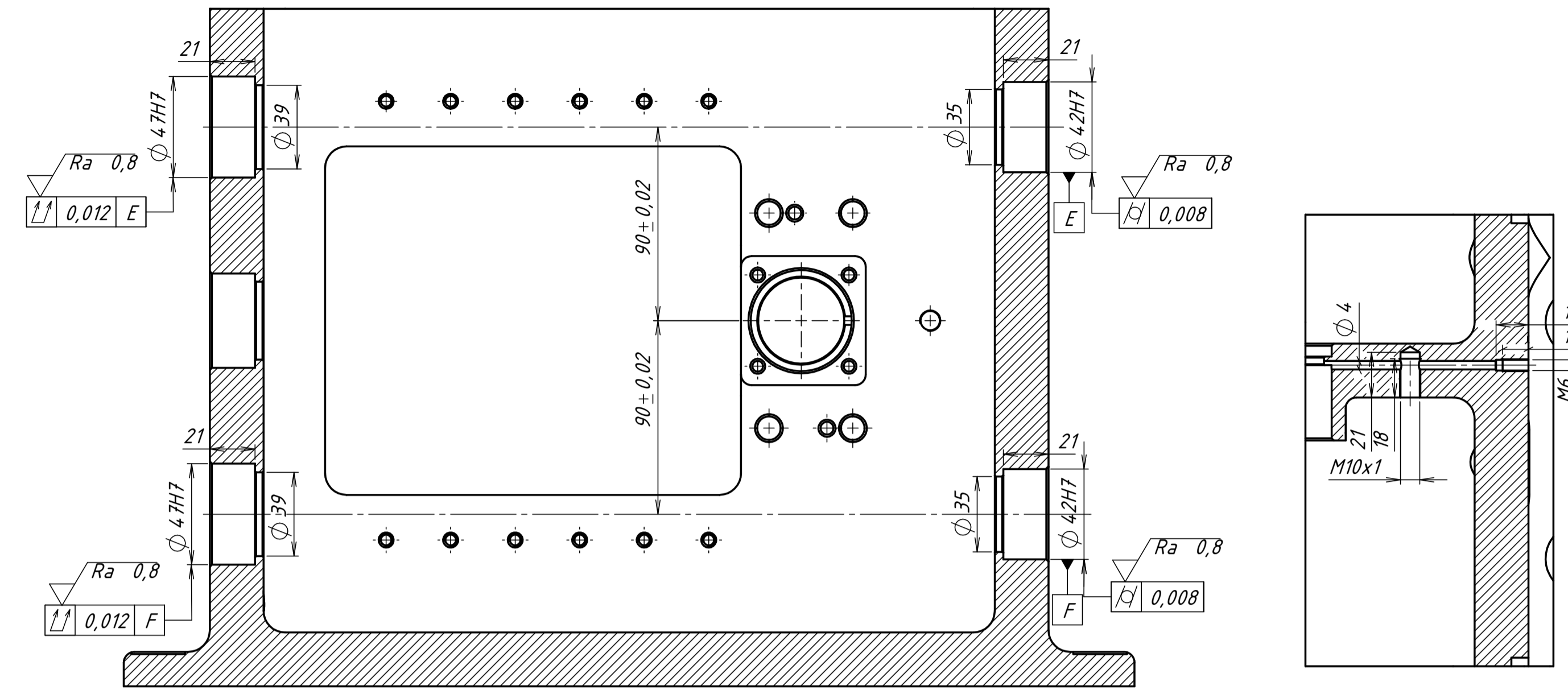
PRESJEK D-D MJERILO 1 : 2
