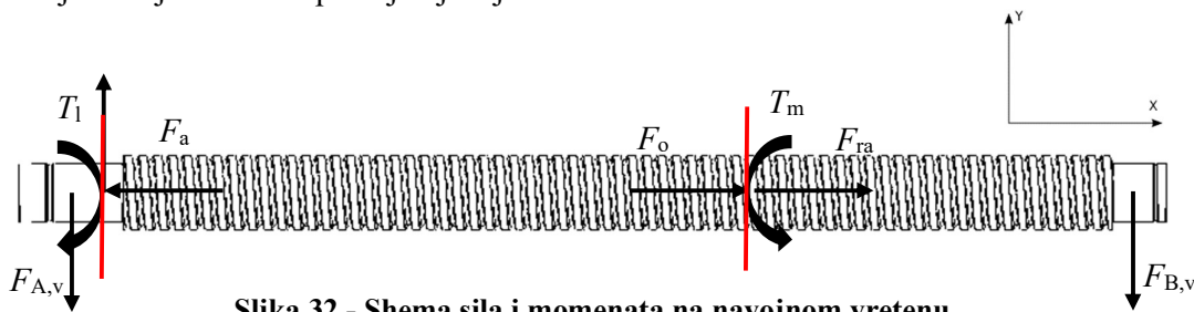
Slika 32 - Shema sila i momenata na navojnom vretenu
