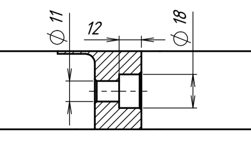
PRESJEK F-F MJERILO 1 : 2
