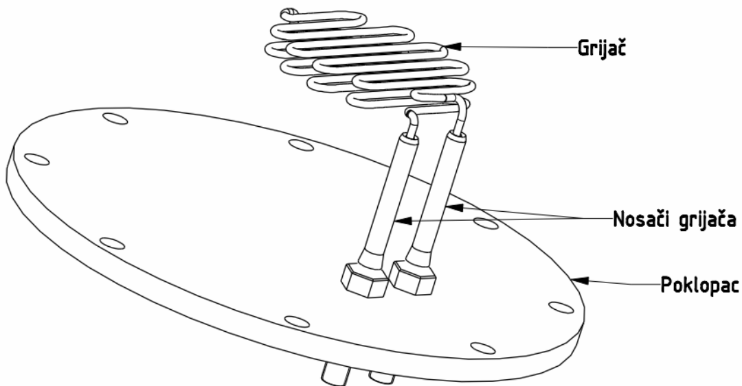
Slika 21. Električni grijač
