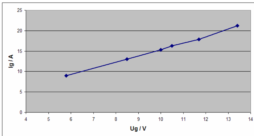
Slika 23. Ovisnost struje kroz grijač o naponu dovedenom na njegove krajeve
