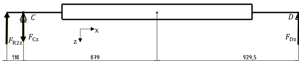
Slika 92. Opterećenje sklopa bubnja u x-z ravnini
