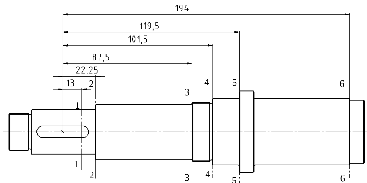
Slika 95. Oblikovano gonjeno vratilo sklopa bubnja
