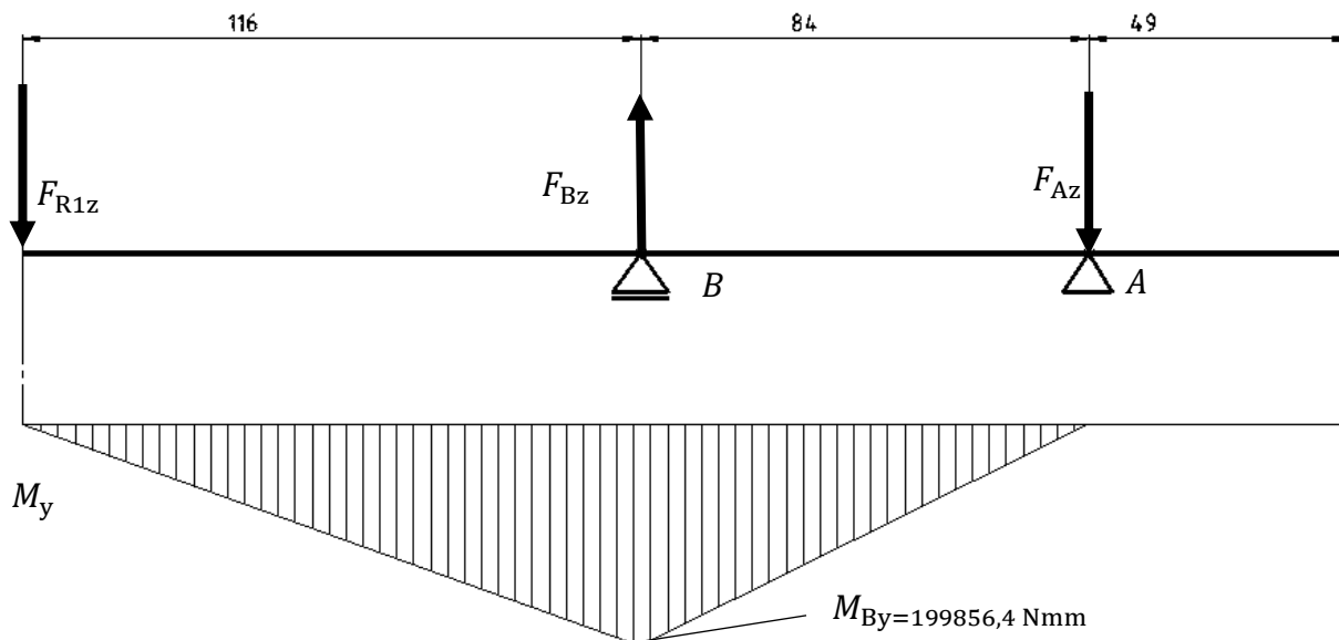
Slika 88. Dijagram momenta svajanja pogonskog vratila u x-z ravni
