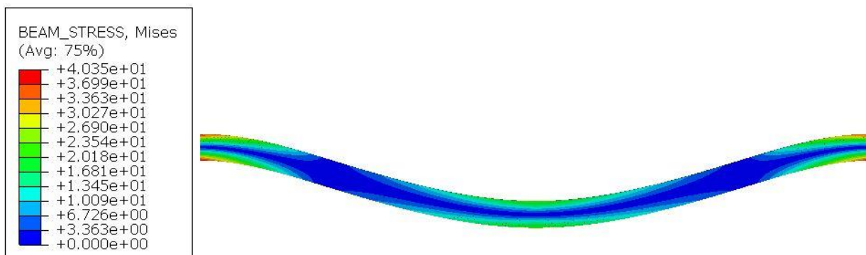
Slika 125. Naprezanja po Von Misesu u naslonu spremnika
