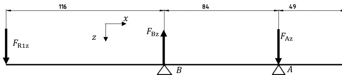
Slika 86. Opterećenje pogonskog vratila u x-z ravnini
