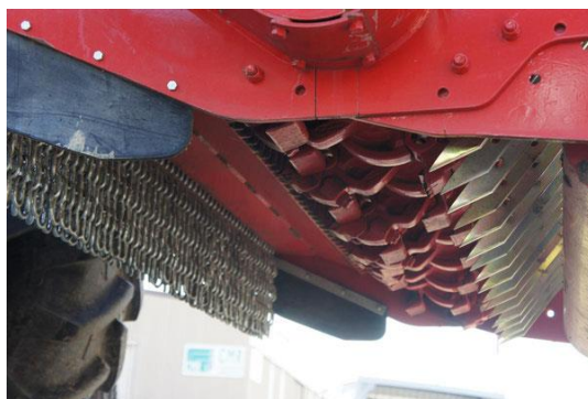
Slika 63. Rotor malčera Midiforst [35]
