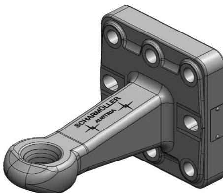
Slika 136. Vučno okno [56]
