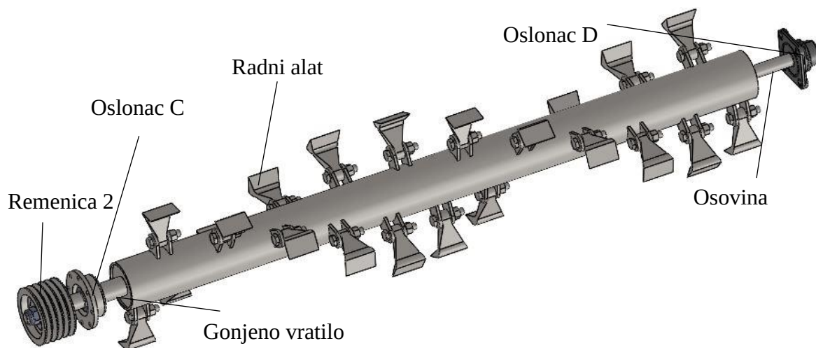
Slika 143. Sklop bubnja
