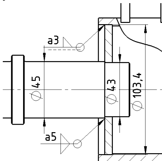
Slika 98. Kritični zavori bubnja
