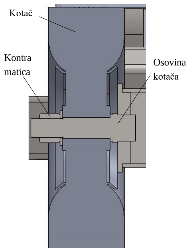
Slika 149. Kotač
