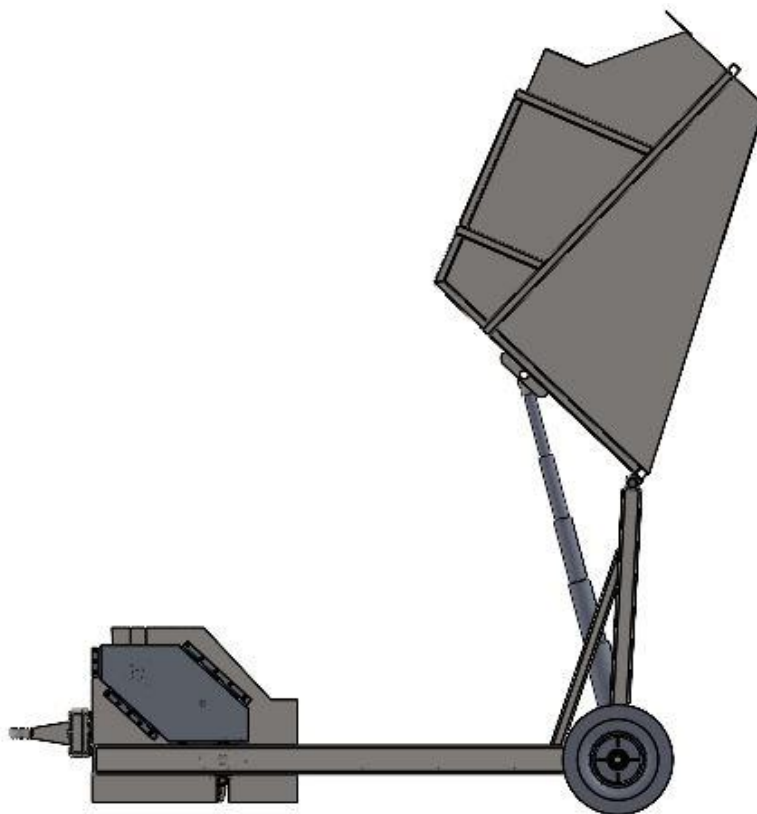
Slika 147. Uređaj prilikom istresanja prikupljanje mase
