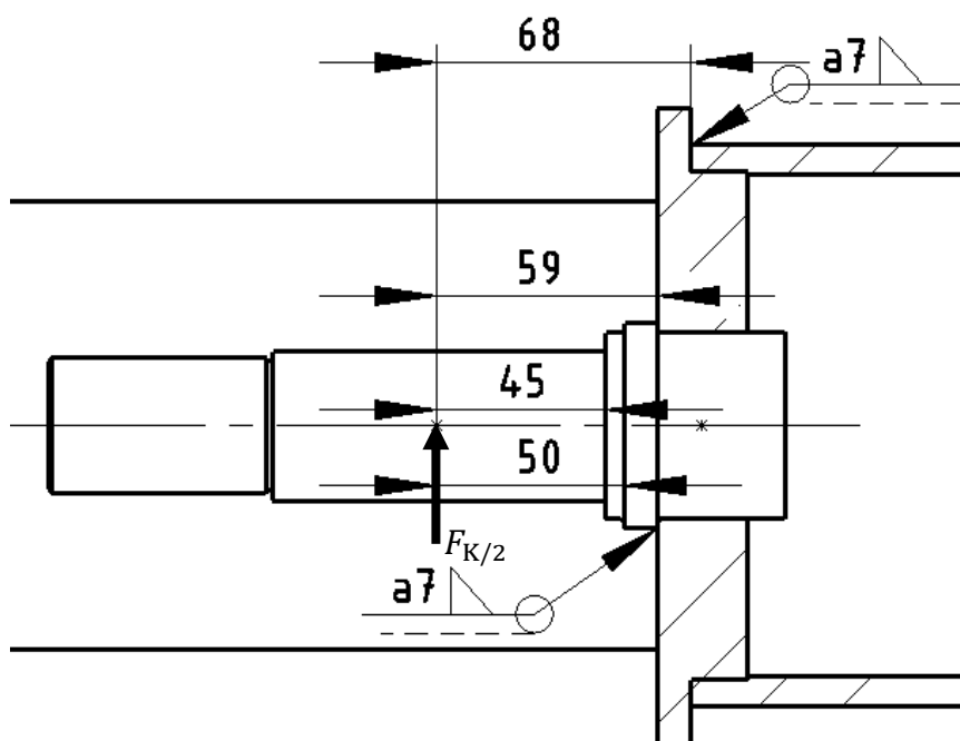
Slika 130. Opterećenje osovine kotača
