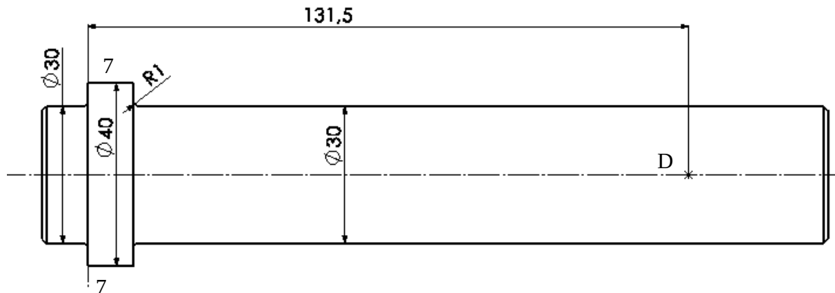
Slika 96. Osovina bubnja
