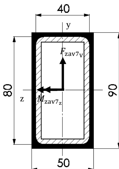
Slika 113. Poprečni presjek zavora 7
