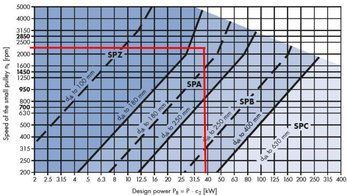
Slika 79. Odabir profila remena [39]
