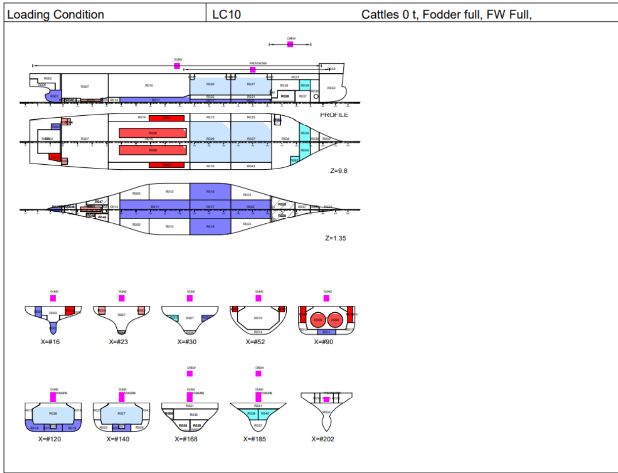
Slika 10. Stanje krcaja koje izaziva minimalni pregibni moment na mirnoj vodi [10]
