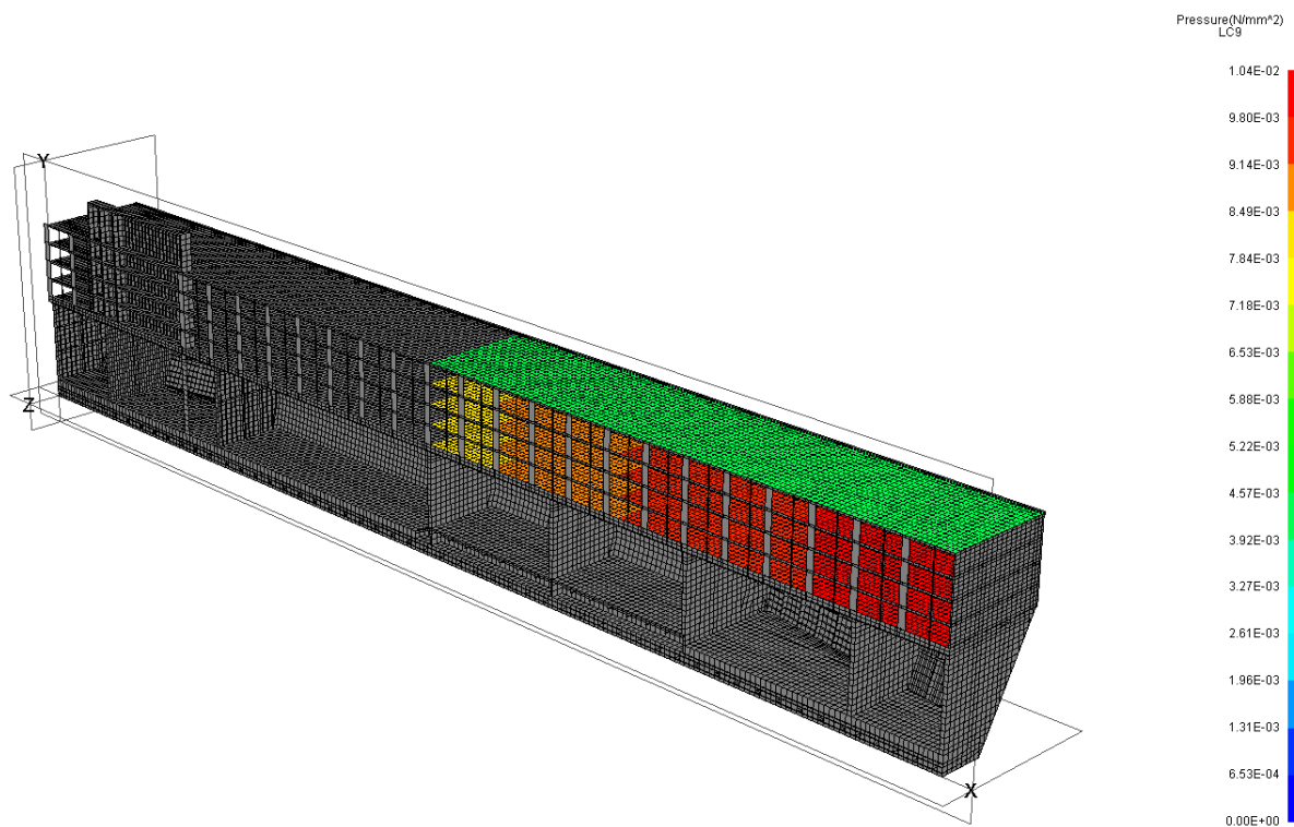
Slika 27. Opterećenja paluba
