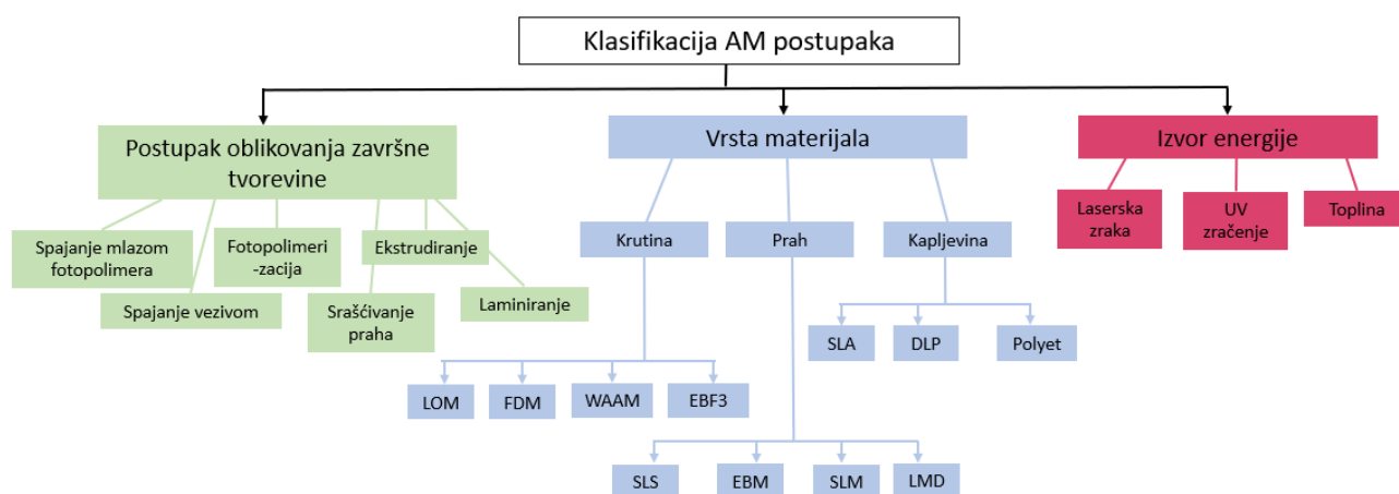
Slika 2.2. Klasifikacija aditivnih postupaka proizvodnje [2]
