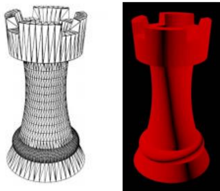
Slika 4.3. STL datoteka s pripadajućom izrađenom tvorevinom [10]
