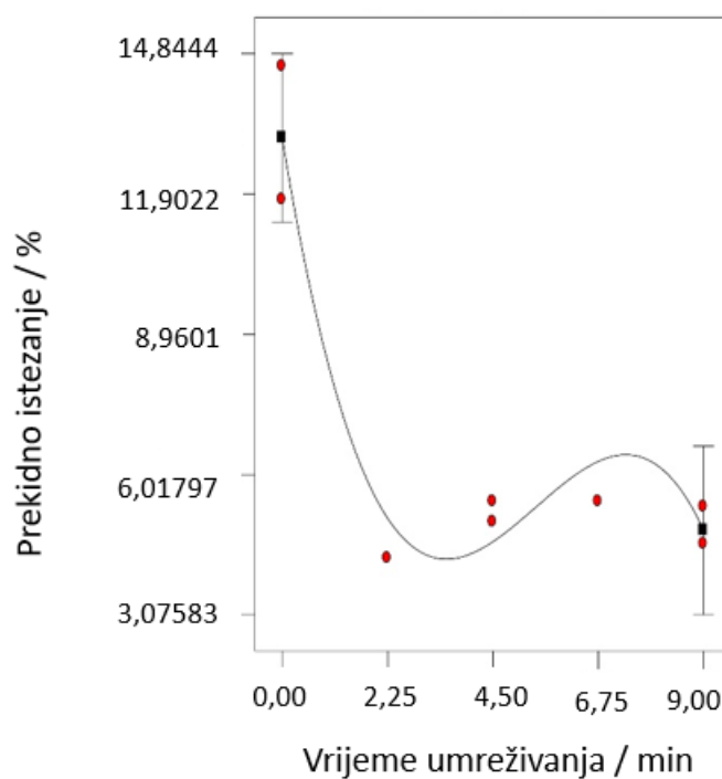
Slika 5.26. Dijagram utjecaja vremena naknadnog umreživanja na prekidno istežanje
