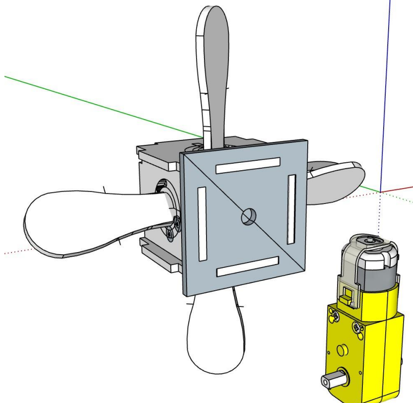
Slika 15. Lopatice robotskog ventilatora
