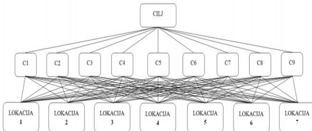
Slika 6. AHP [2]
