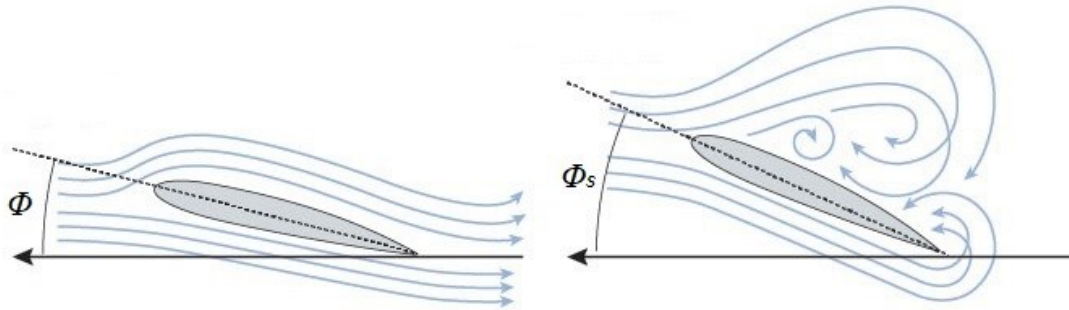
Slika 4.2. Aerodinamički zastoј [16]
