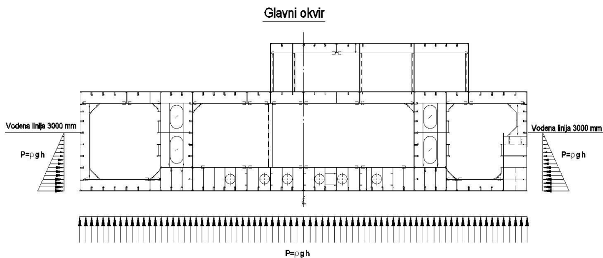
Slika 4.3-1 Hidrostatski tlak
