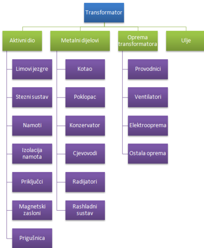
Slika 29. Komponente transformatora
