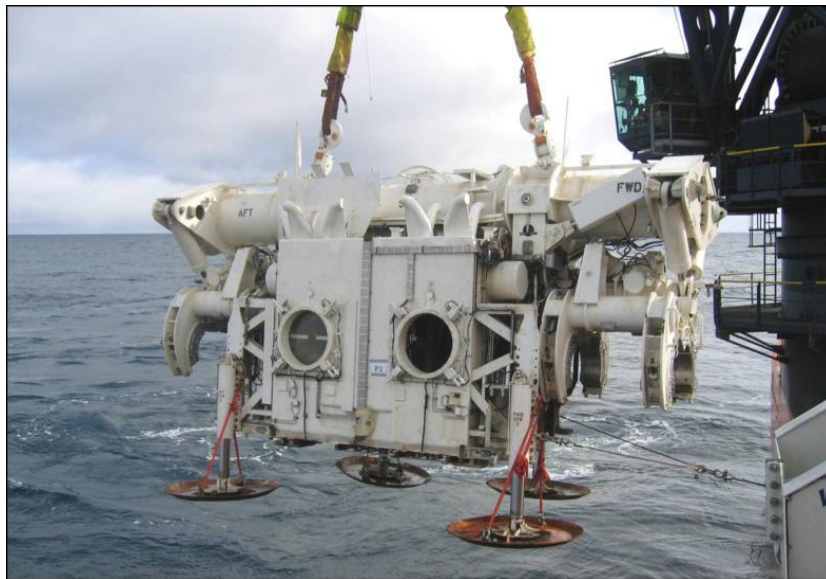
Slika 4.15 Zavarivačka komora PRS welding habitat [56]
