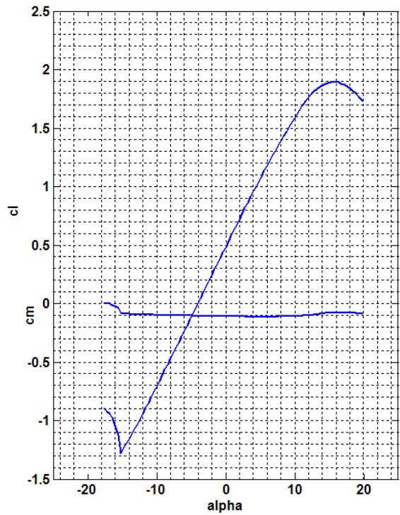
Slika 28 Polara za ONERA 12 aeroprofil
