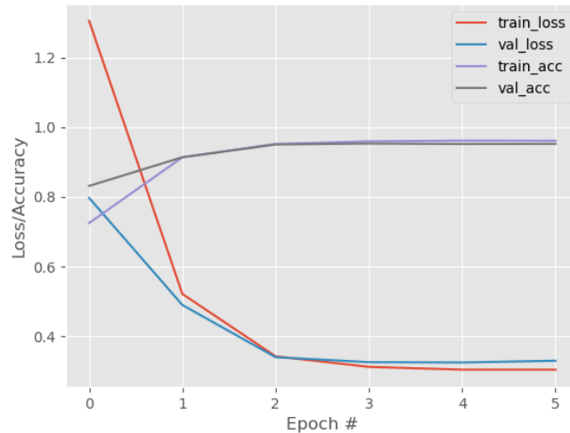
Slika 5.11 Gubitak i točnost kao funkcije broja epoha kod modela za slike iz kadra HE, eksperiment 2
