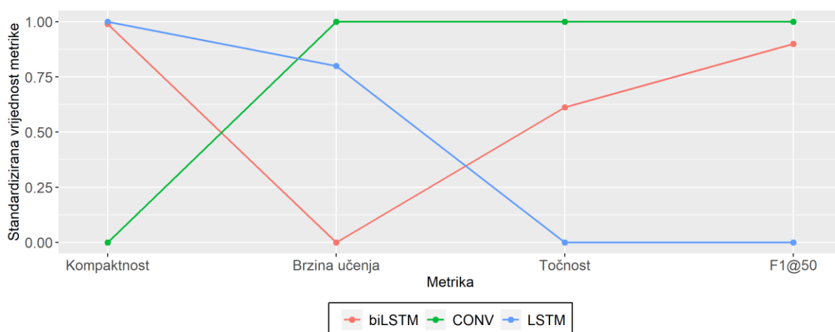
Slika 5.43 Standardizirane vrijednosti 4 metrike kod modela za kadar HE i pristup TB
