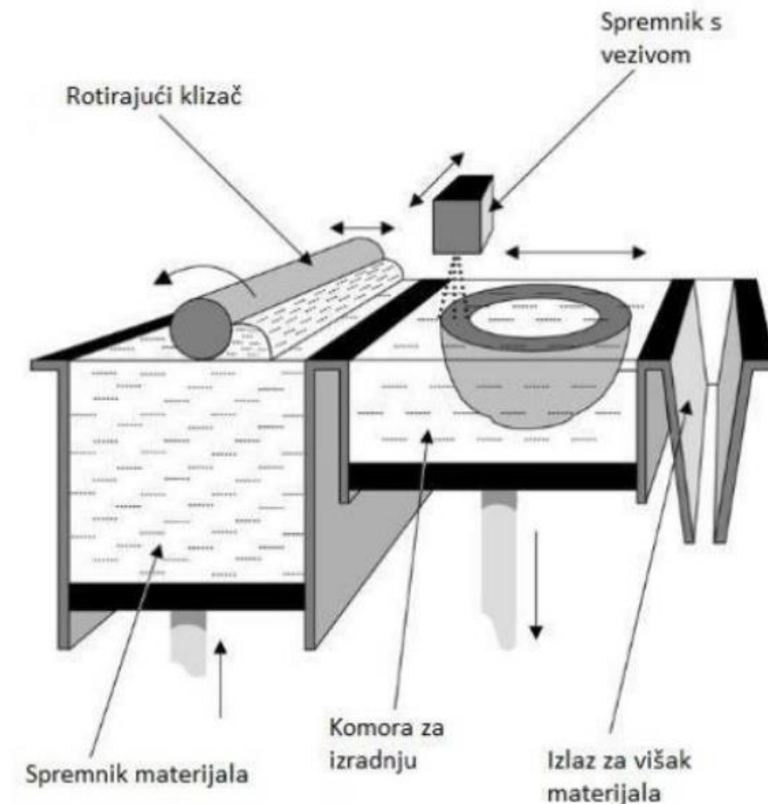
Slika 3. Prikaz 3DP postupka [4]
