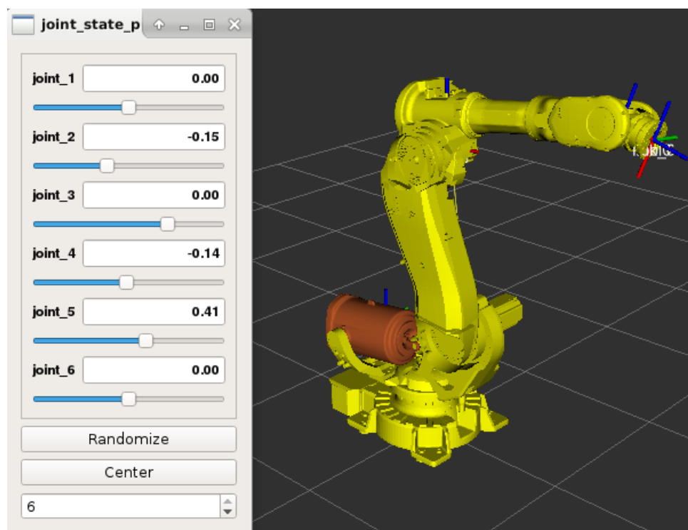
Slika 34 Uspješna vizualizacija modela robota u RViz-u
