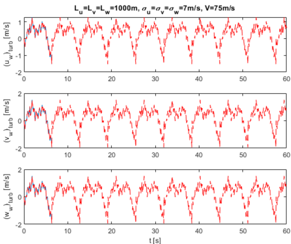
Slika 26. Komponente turbulentnog vektora brzine vjetra u ponavljajućoj sekvenci
