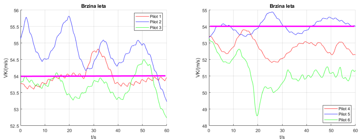
Slika 47. Prikaz brzina leta tijekom simulacije (zadatak 3)
