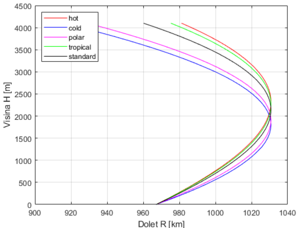
Slika 13. Raspon doleta zrakoplova za odabrane atmosfere
