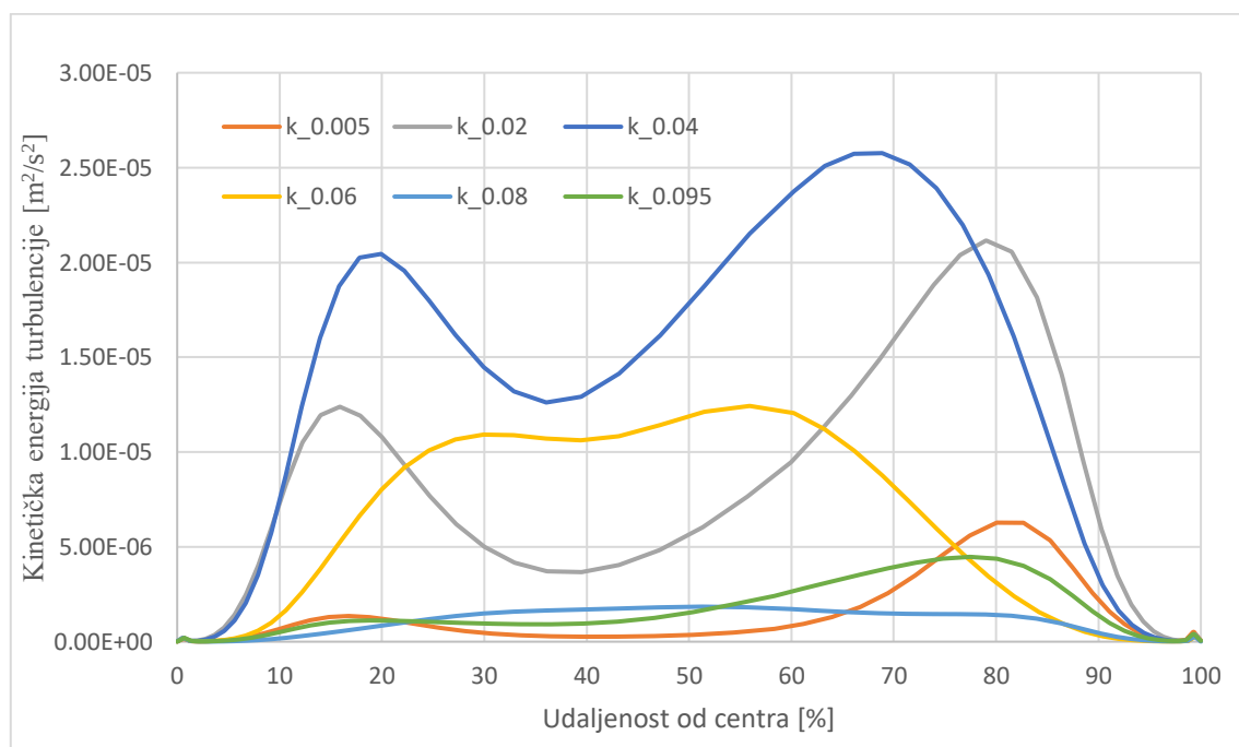
Slika 54. Radijalna raspodjela kinetičke energije turbulencije u lažnom lumenu po presjecima u t=9.47\text{s}
