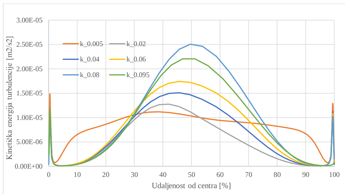
Slika 47. Radijalna raspodjela kinetičke energije turbulencije u stvarnom lumenu po presjecima u t=9.17\text{s}
