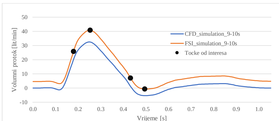
Slika 12. Usporedba protoka dobivenih CFD i FSI simulacijama u lažnom lumenu sa naznačenim točkama od interesa
