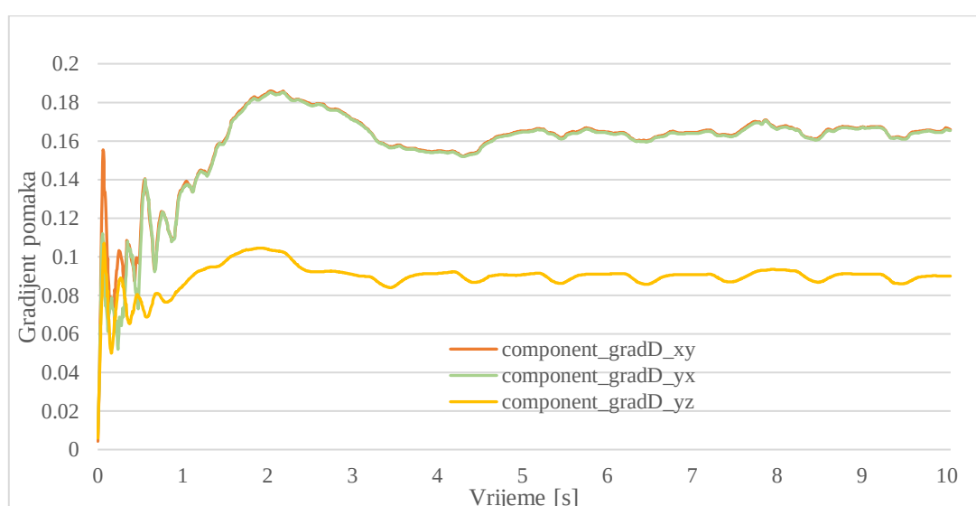
Slika 59. Komponente maksimalnog gradijenta pomaka sa najvećim oscilacijama
