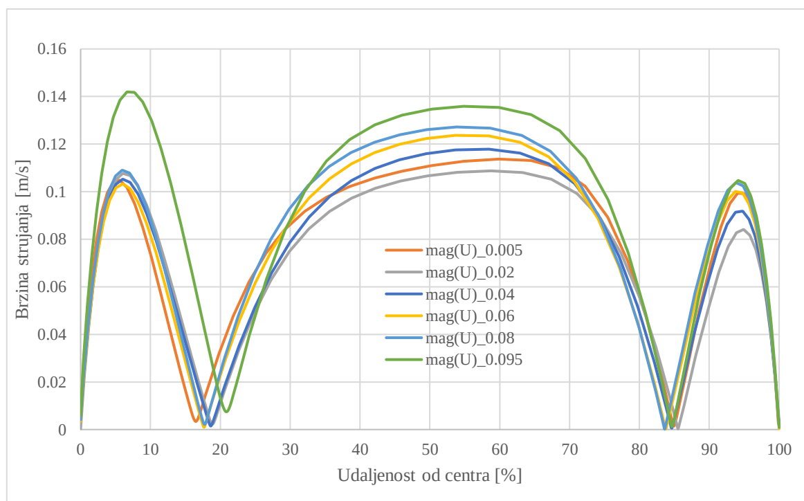
Slika 43. Radikalna raspodjela brzine strujanja u stvarnom lumenu po presjecima u t=9.41s
