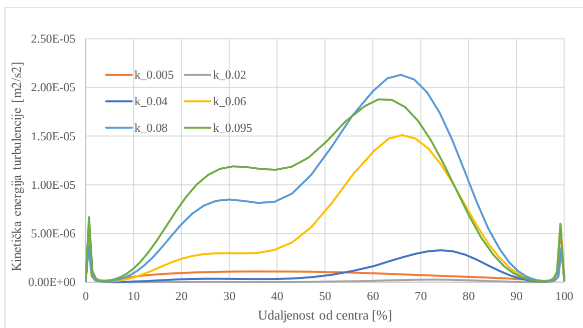
Slika 48. Radijalna raspodjela kinetičke energije turbulencije u lažnom lumenu po presjecima u t=9.17\text{s}
