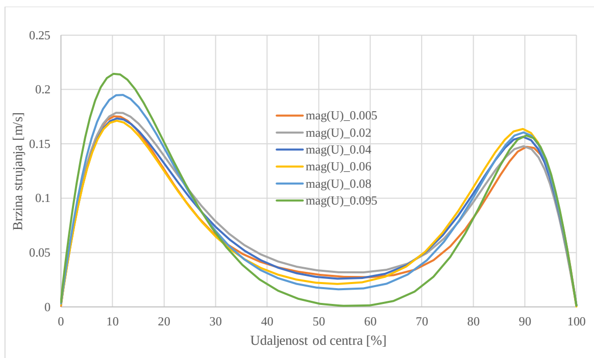
Slika 45. Radijalna raspodjela brzine strujanja u stvarnom lumenu po presjecima u t=9.47\text{s}
