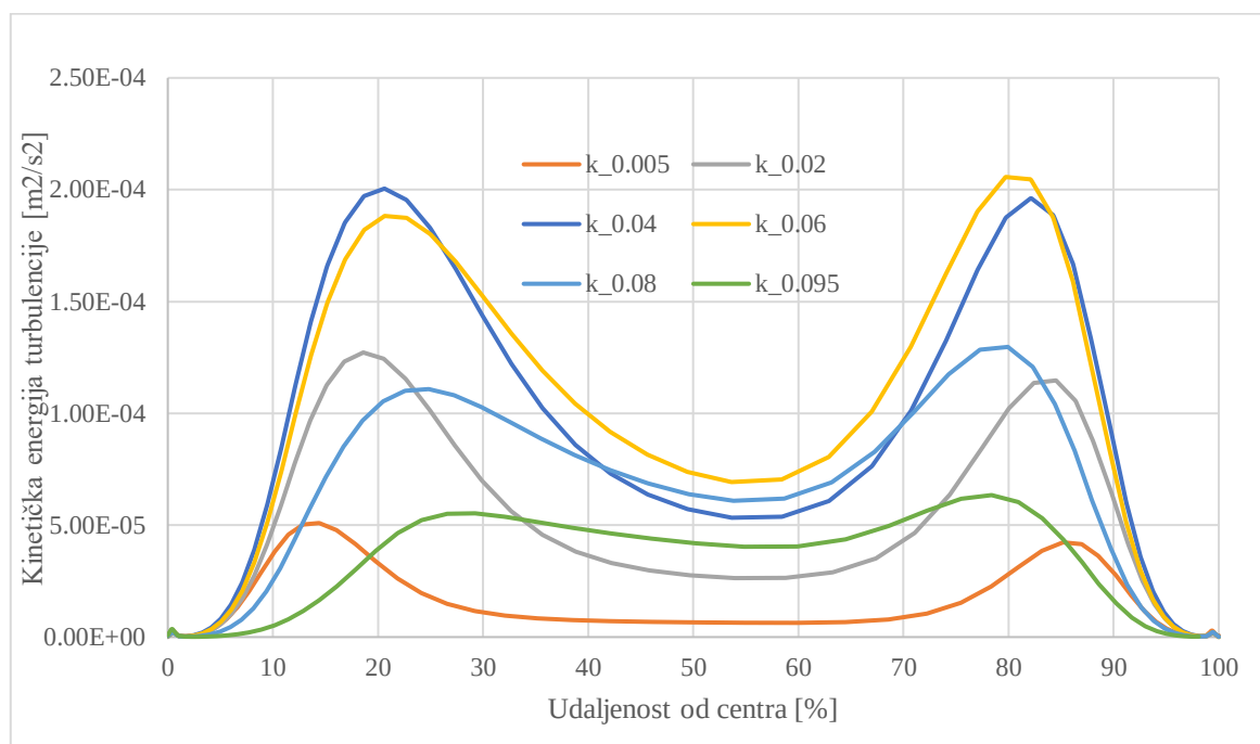
Slika 51. Radijalna raspodjela kinetičke energije turbulencije u stvarnom lumenu po presjecima u t=9.41\text{s}
