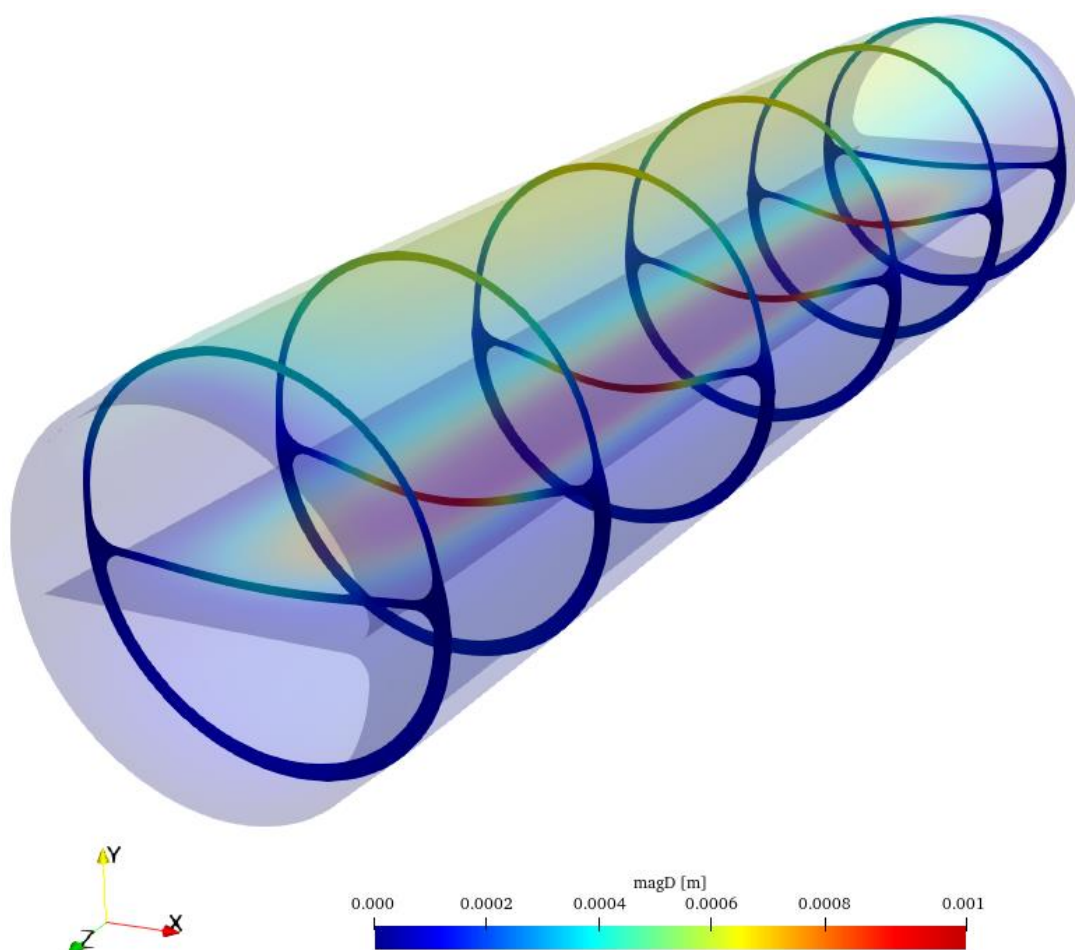
Slika 60. Prikaz deformirane aorte sa presjecima u trenutku maksimalnog tlaka u t=9.17s
