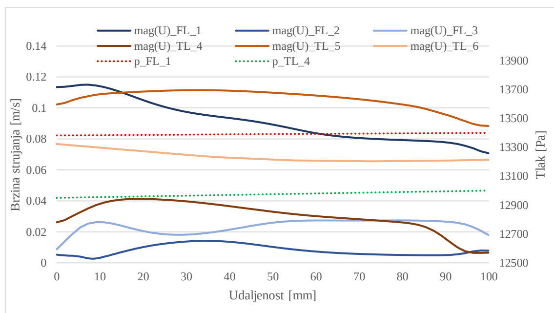
Slika 34. Brzina strujanja i tlak duž aorte u t=9.47s
