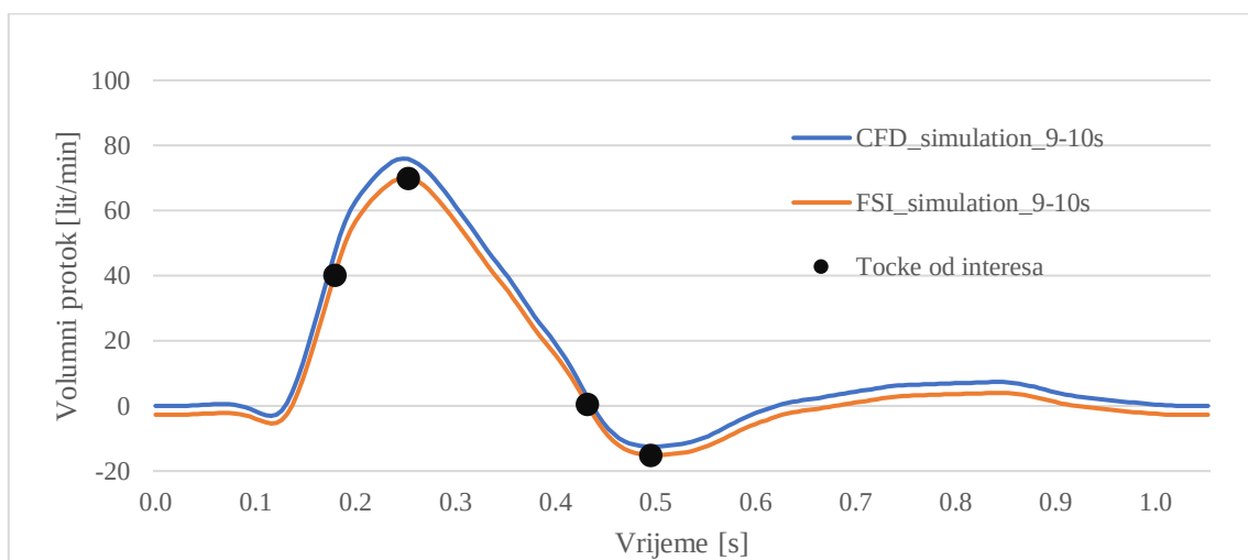
Slika 11. Usporedba protoka dobivenih CFD i FSI simulacijama u stvarnom lumenu sa naznačenim točkama od interesa
