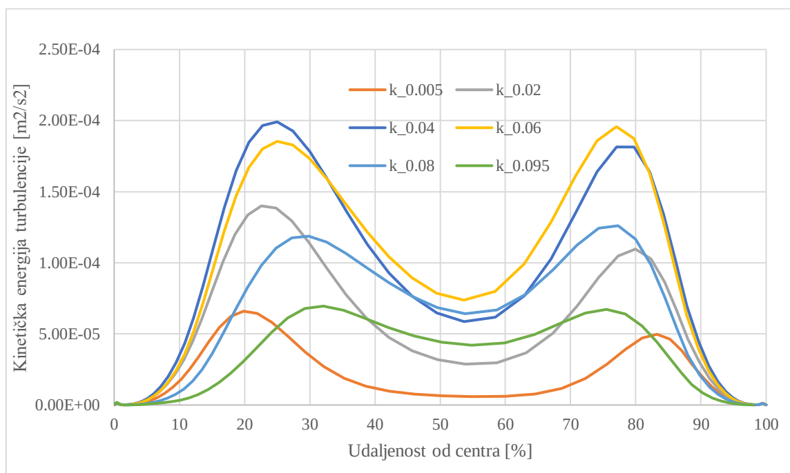
Slika 53. Radijalna raspodjela kinetičke energije turbulencije u stvarnom lumenu po presjecima u t=9.47\text{s}
