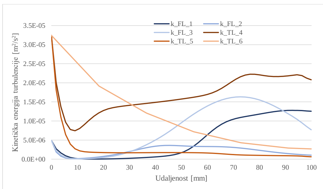
Slika 35. Kinetička energija turbulencije duž aorte u t=9.17\text{s}
