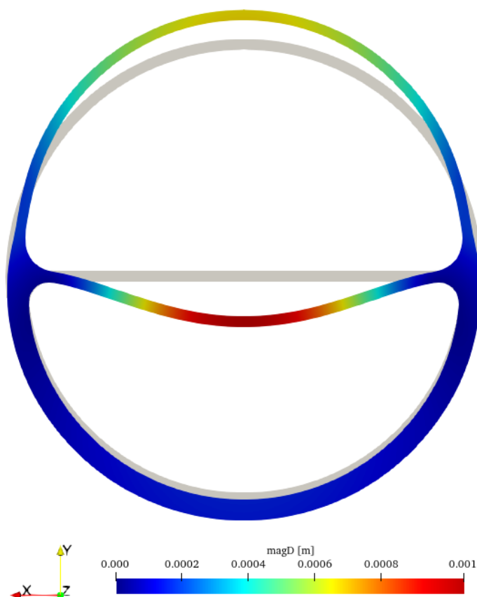
Slika 61. Raspodjela pomaka na poprečnom presjeku na sredini domene
