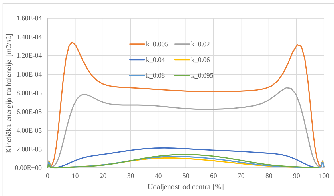
Slika 49. Radijalna raspodjela kinetičke energije turbulencije u stvarnom lumenu po presjecima u t=9.24\text{s}
