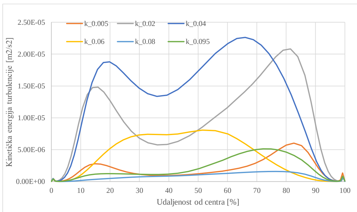
Slika 52. Radijalna raspodjela kinetičke energije turbulencije u lažnom lumenu po presjecima u t=9.41\text{s}
