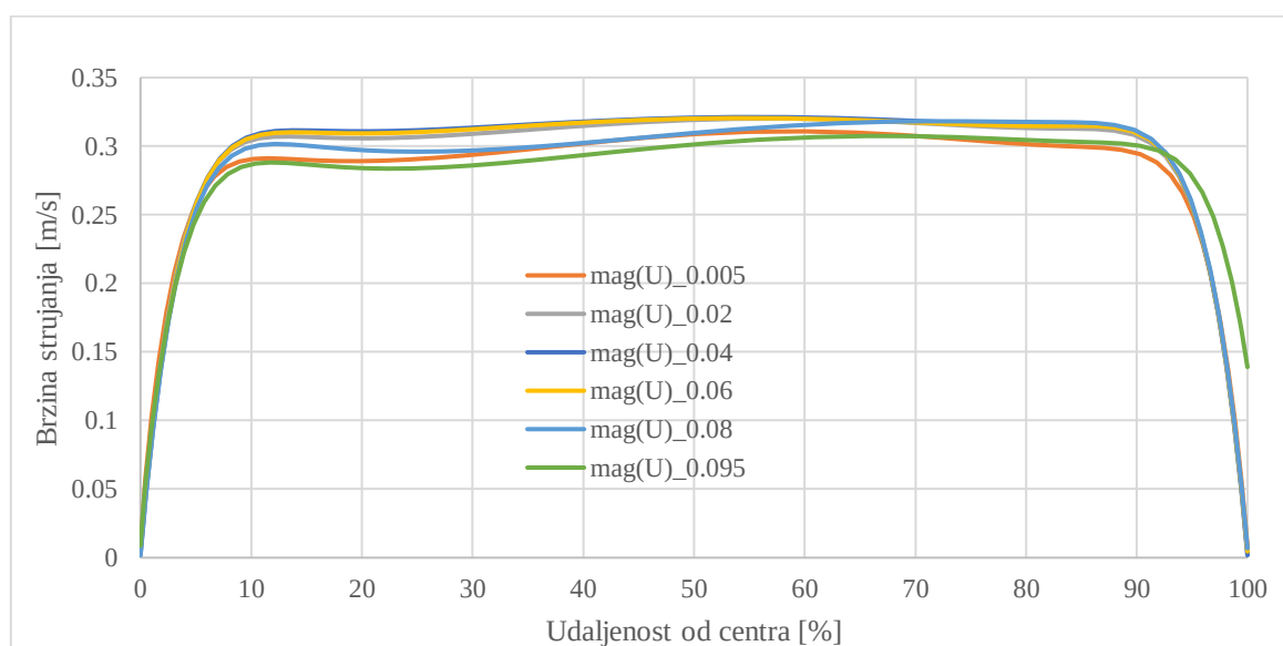
Slika 39. Radijalna raspodjela brzine strujanja u stvarnom lumenu po presjecima u t=9.17s
