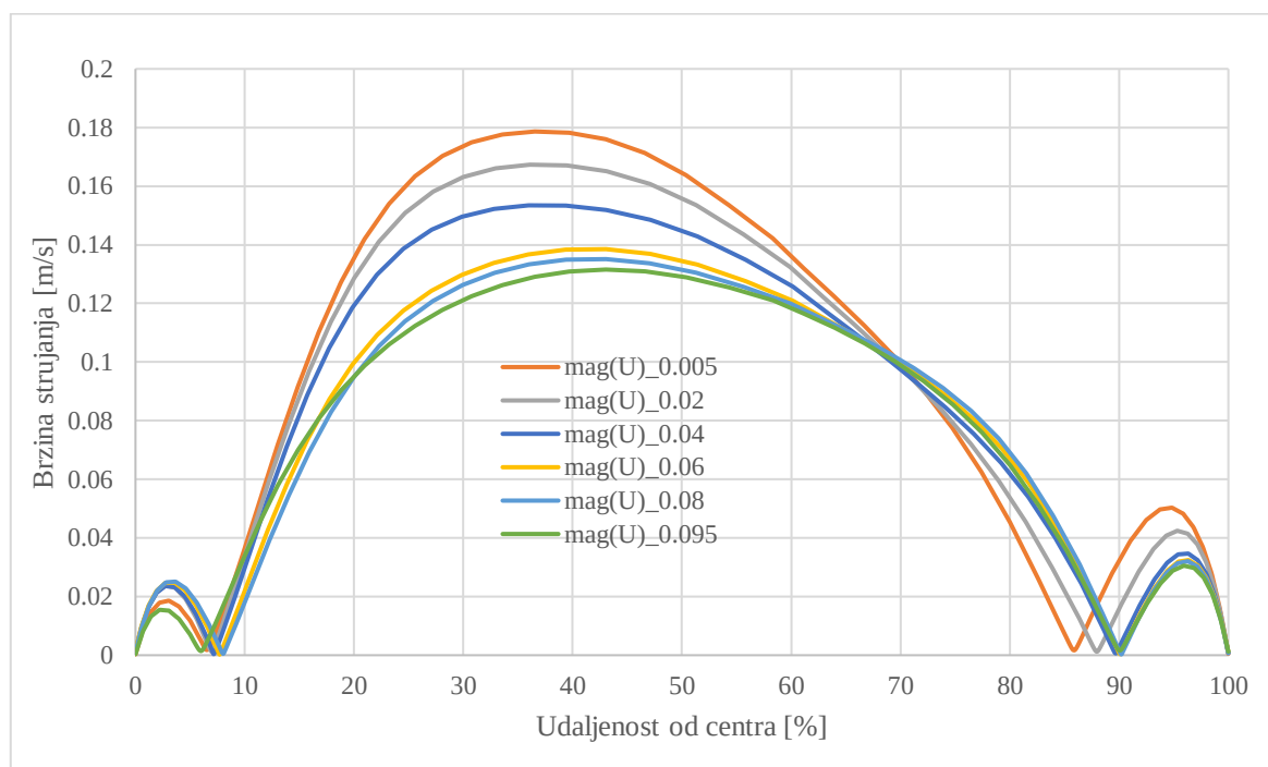
Slika 44. Radijalna raspodjela brzine strujanja u lažnom lumenu po presjecima u t=9.41\text{s}
