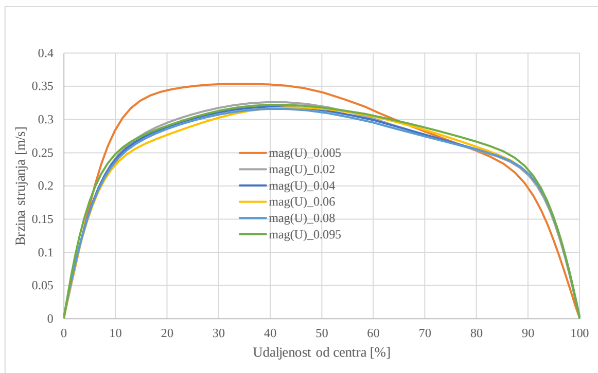
Slika 42. Radikalna raspodjela brzine strujanja u lažnom lumenu po presjecima u t=9.24s
