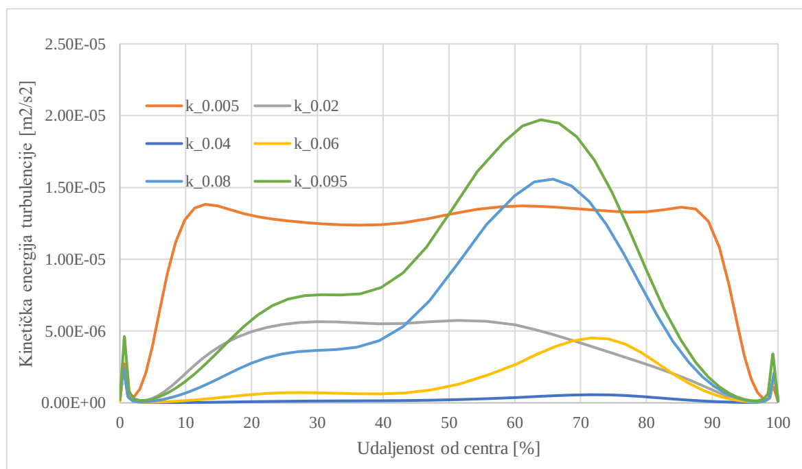
Slika 50. Radijalna raspodjela kinetičke energije turbulencije u lažnom lumenu po presjecima u t=9.24\text{s}
