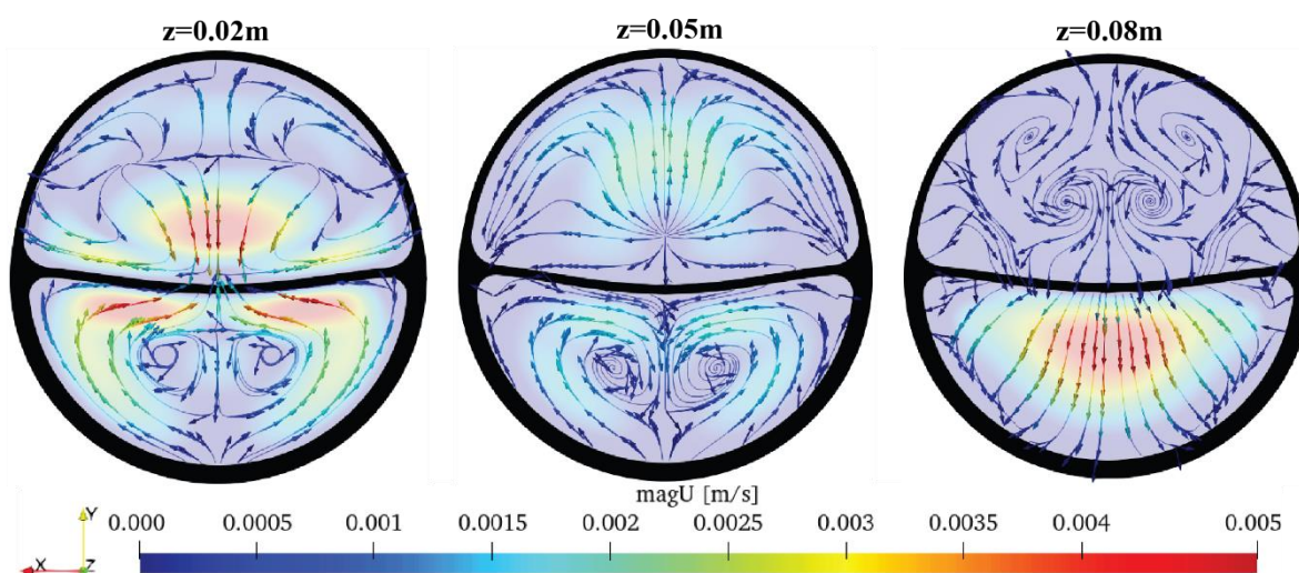
Slika 20. Prikaz brzine strujanja po poprečnim presjecima u t=9.47s
