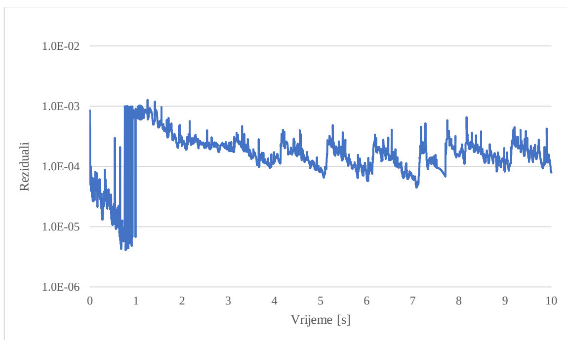
Slika 56. FSI reziduali
