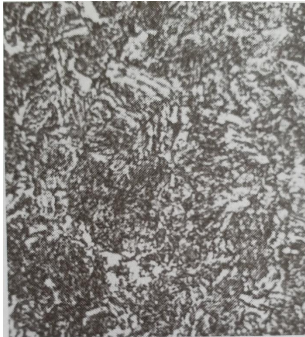
Slika 76. Primjer mikrostrukture iz literature -42CrMo4 čelična šipka, austenitizirano na 845°C, kaljeno u ulju na 65°C i žareno dva sata pri na 620°C. Struktura je mješavina martenzita, ferita i karbida. Uzorak je nagrižen 2% - tnom otopinom nitala, povećanje 750x[11]
