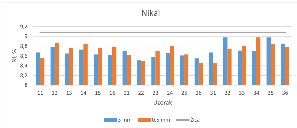
Slika 53. Udio nikla
