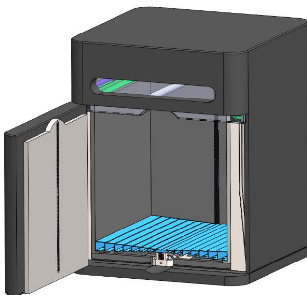
Slika 17 SLS uređaj [29]
