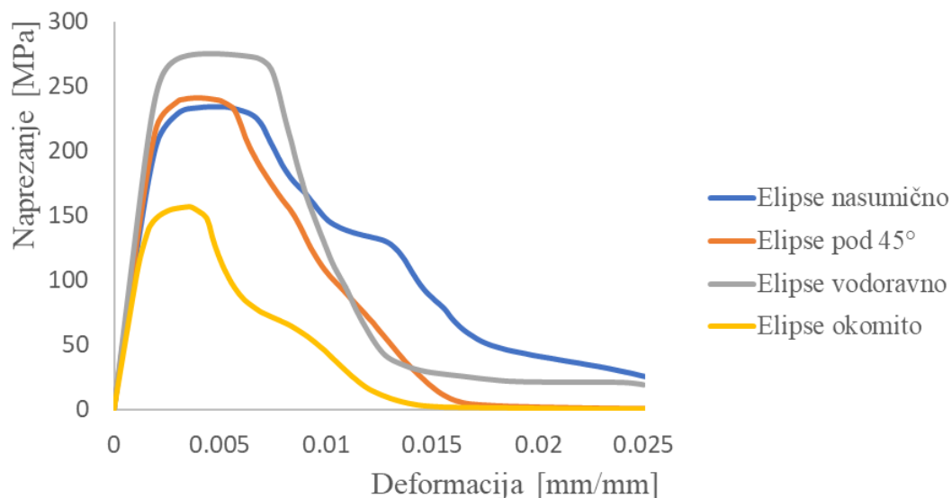
Slika 49. \sigma - \epsilon dijagram usporedbe položaja nepravilnosti u obliku elipsa omjera stranica 1/2
