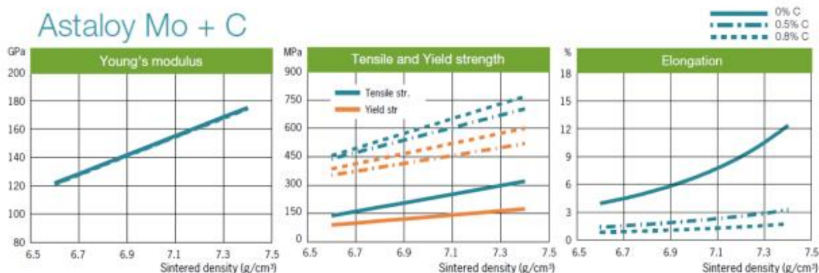
Slika 34. Utjecaj udjela ugljika na Youngov modul elastičnosti, vlačnu čvrstoću, granicu tečenja i istezljivost
