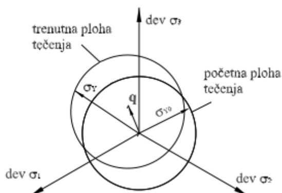
Slika 16. Grafički prikaz kinematičkog očvršćenja [15]
