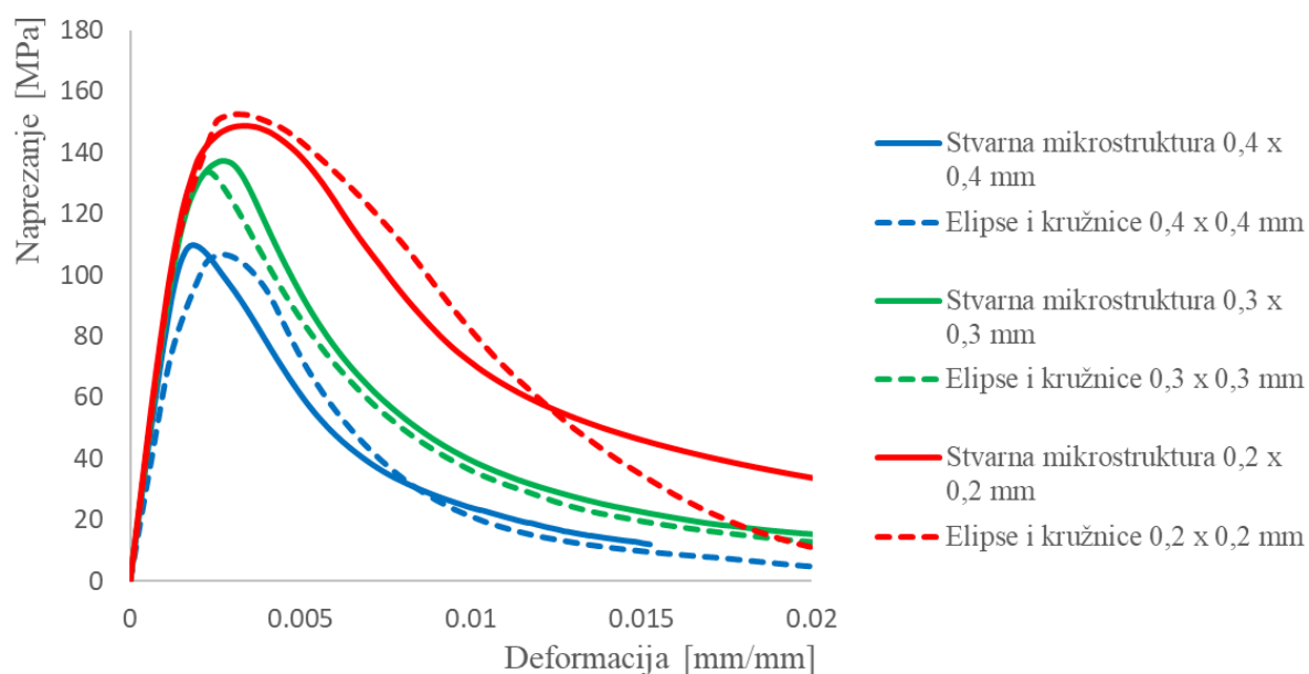
Slika 62. Pogađanje stvarne mikrostrukture
