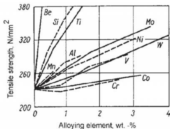
Slika 11. Vlačna čvrstoća u ovisnosti o legiranim elementima u sinteriranom čeliku [9]
