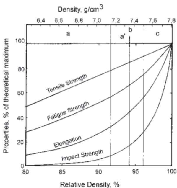
Slika 9. Utjecaj gustoće na mehanička svojstva [9]
