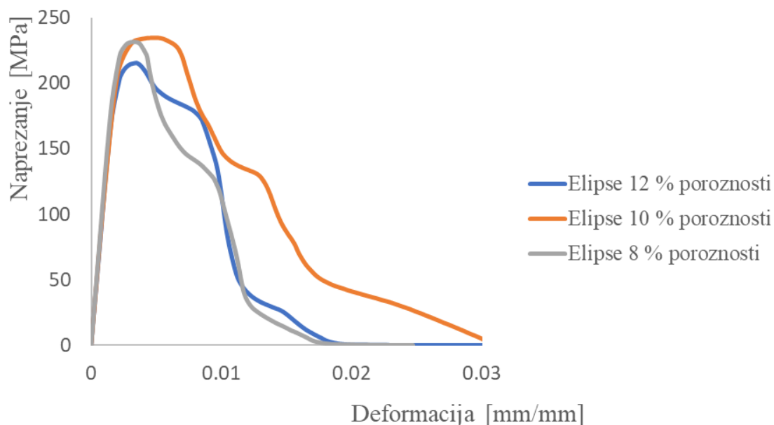
Slika 50. Usporedba \sigma - \epsilon dijagrama za RVE-ove s nasumično postavljenim elipsama omjera stranica 1/2 za 8, 10 i 12 % poroznosti
