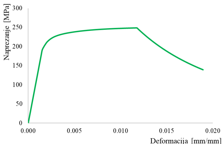
Slika 35. Idealiziran \sigma - \epsilon dijagram na temelju podataka iz literature [9] za sinterirani čelik Astaloy Mo + 0,2C gustoće 6,5 g/cm 3
