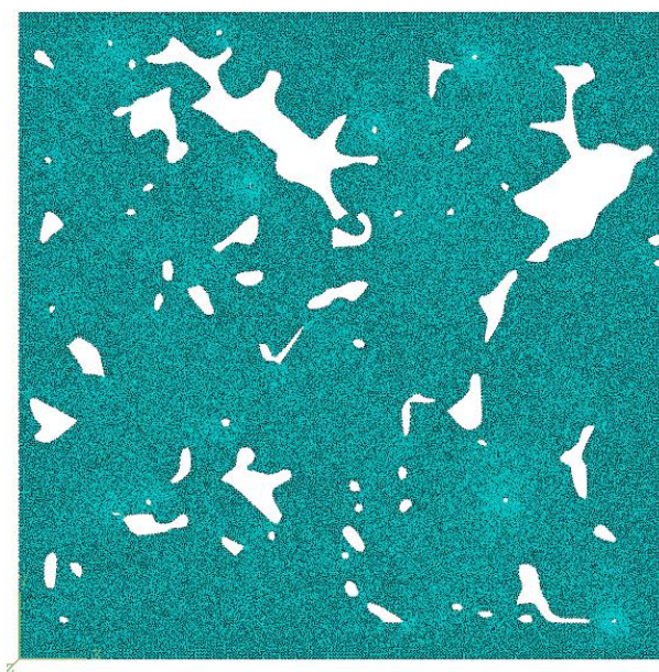
Slika 57. Mreža konačnih elemenata za RVE veličine 0,2 x 0,2 mm
