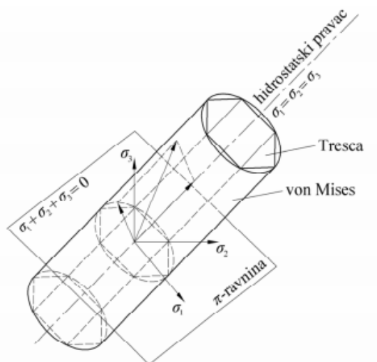
Slika 14. Von Misesova i Trescina ploha tečenja [13]
