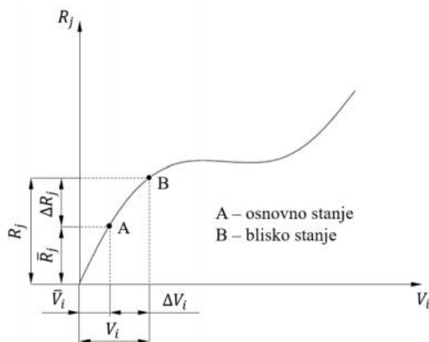
Slika 28. Nelinearna veza između opterećenja i pomaka [5]
